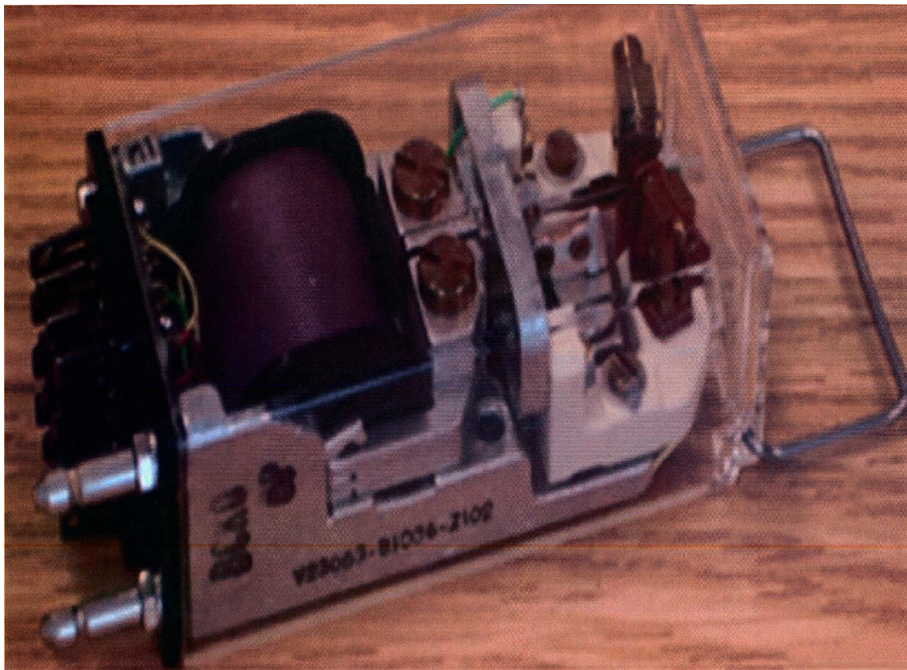
65. Реле (от 1 до 30 штук).
