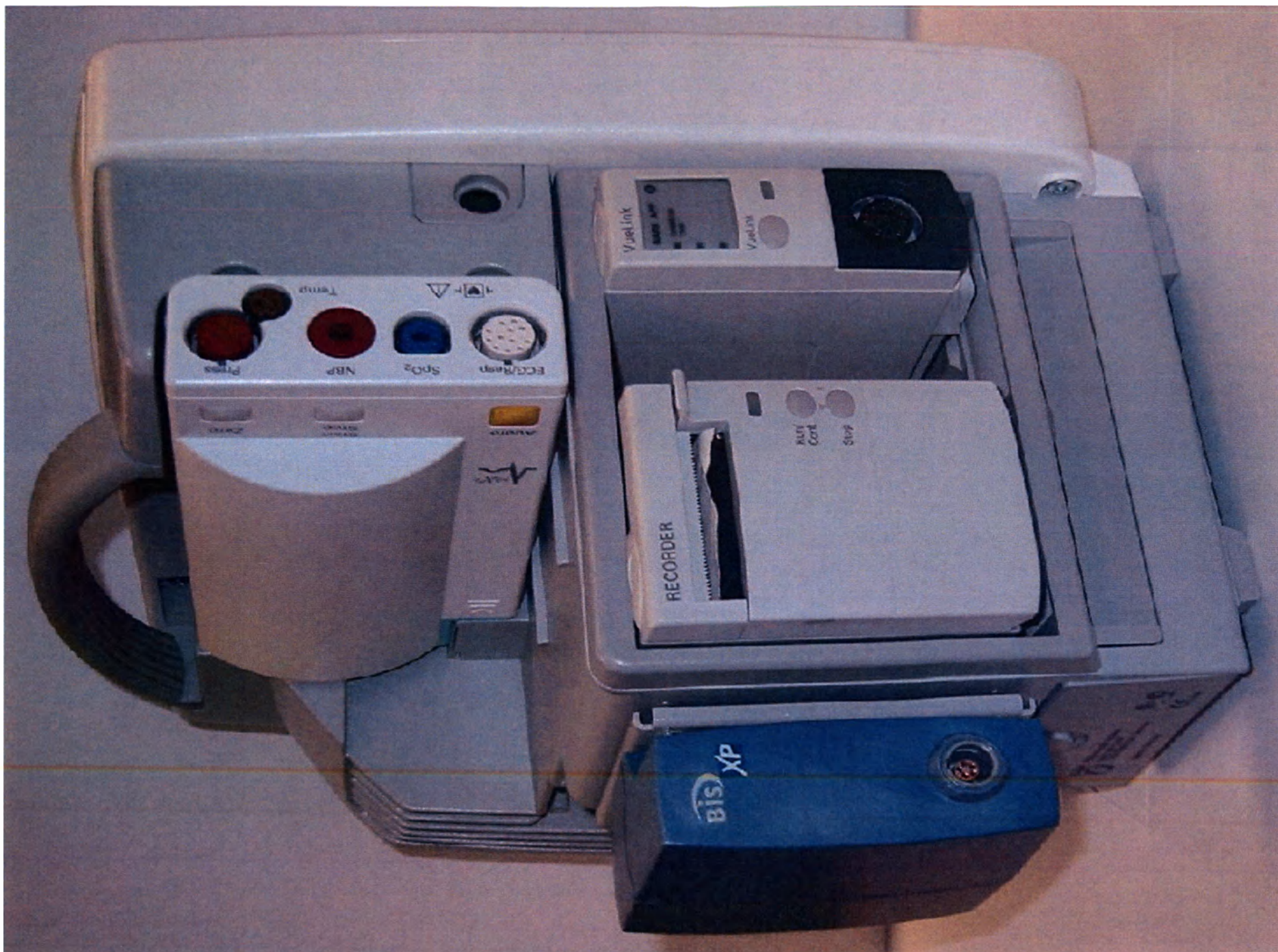
34. Блоки электрофизиологии (от 1 до 5 штук).
