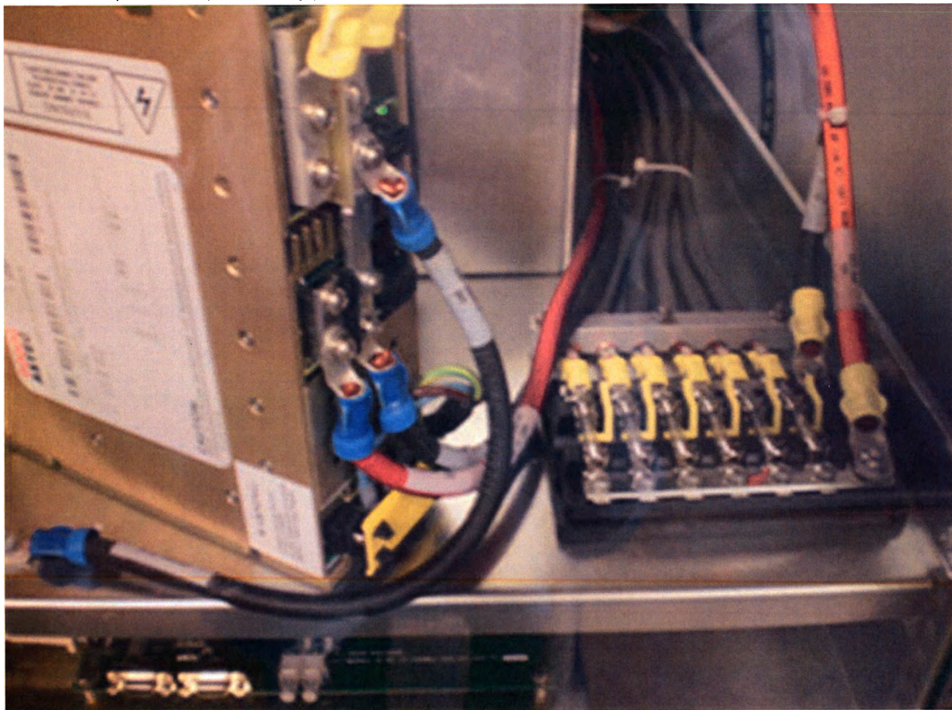
32. Блоки измерения дозы (от 1 до 5 штук).
