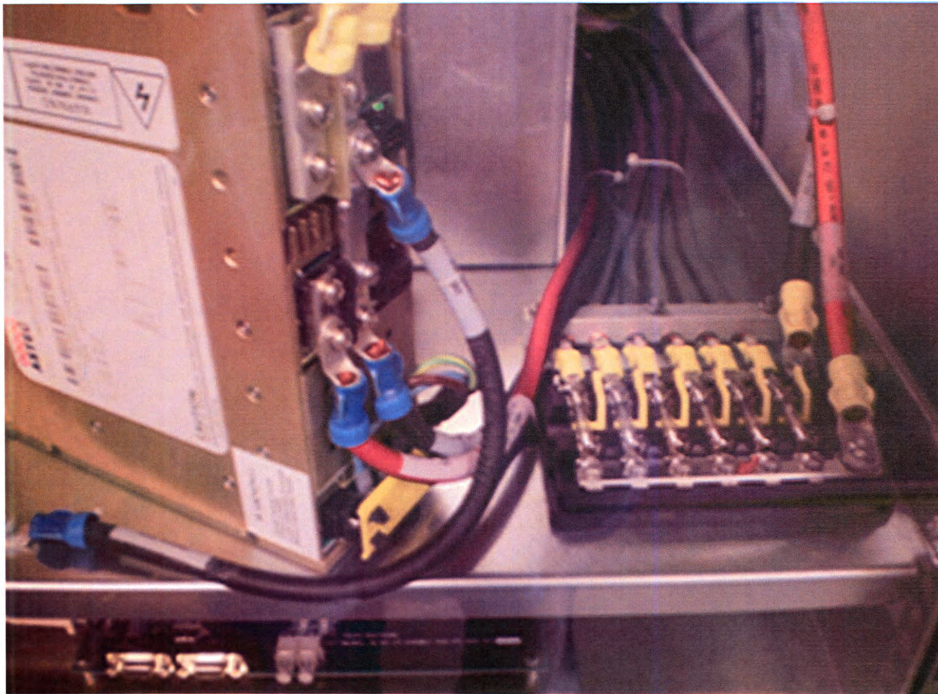
Блоки расчета дозы (от 1 до 5 штук)
