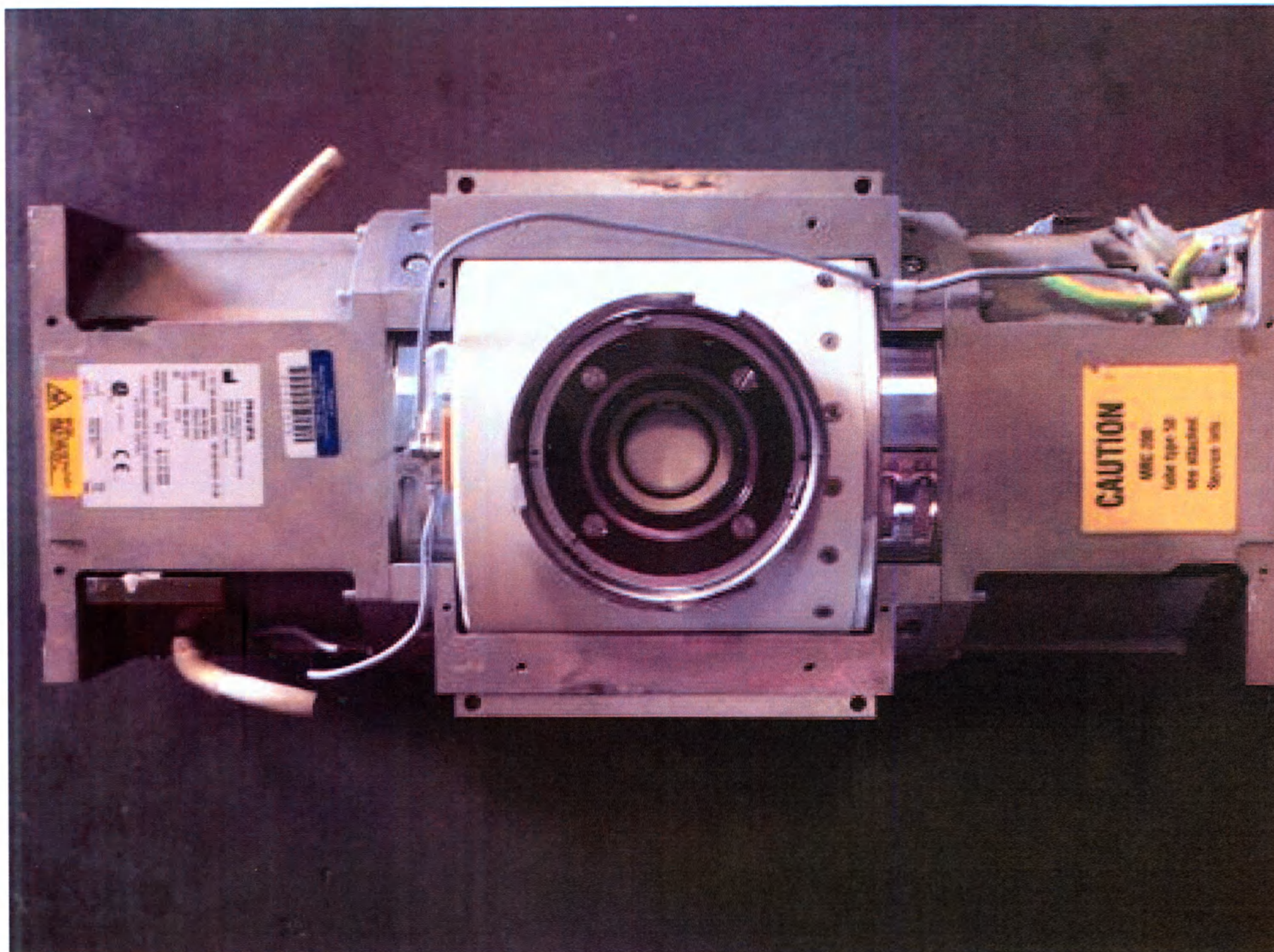
Рентгеновская трубка
