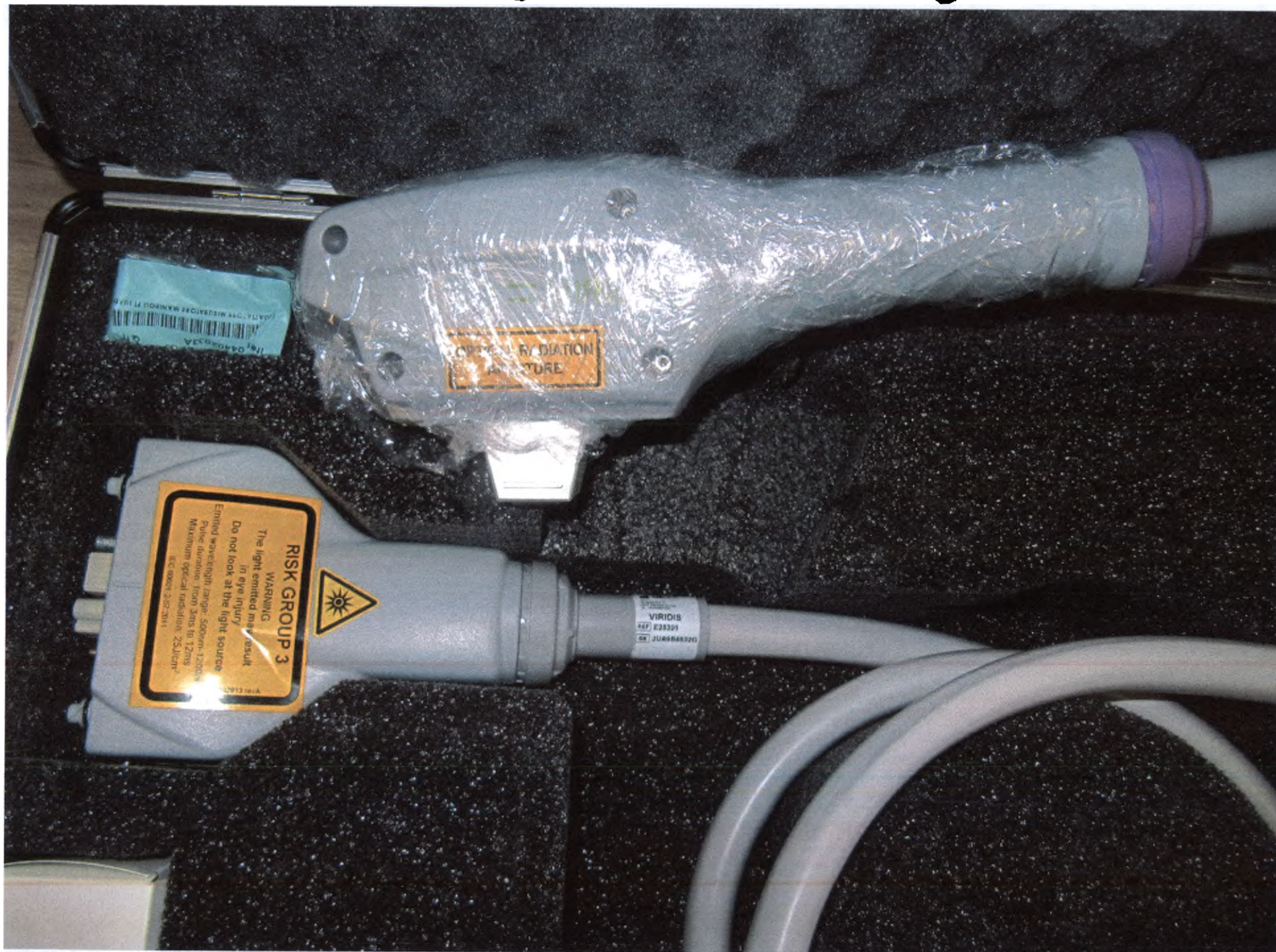
Фото 52 – Маркировка манипулятора Viridis.
