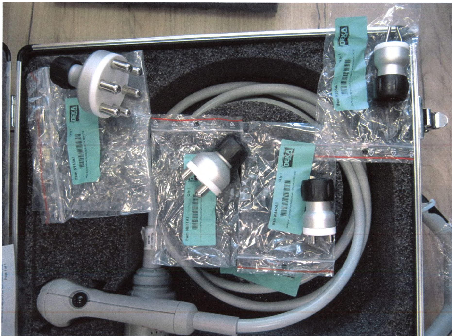
Фото 100 - Наконечники манипулятора Setis: очень маленького размера, среднего размера, большого размера, гексаполярный.
