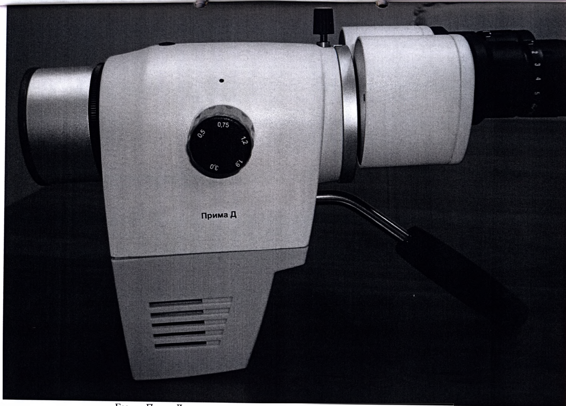
Голова Прима Д с установленными окулярами 10× , объективом 250 и тубусом 90
