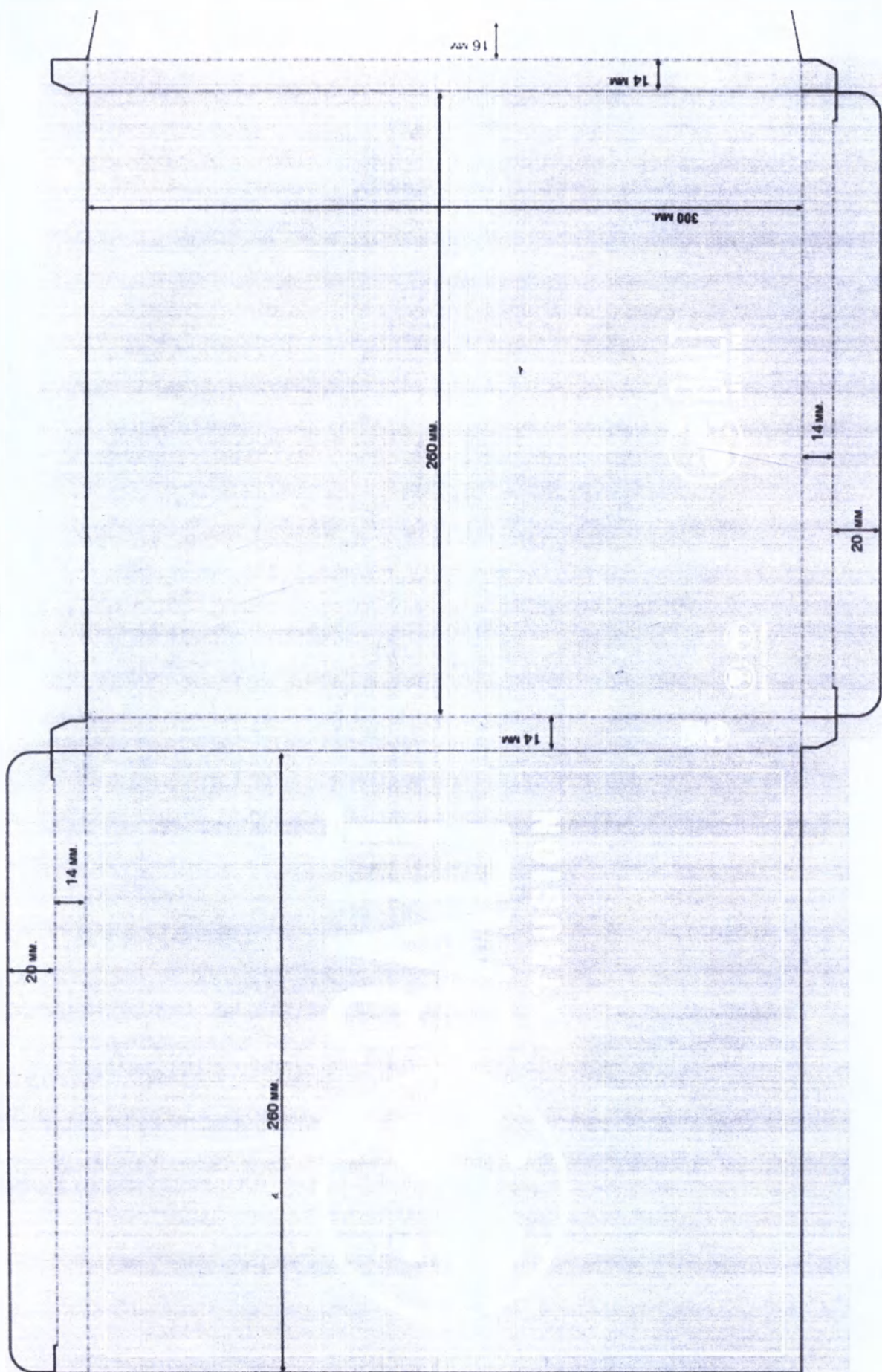
Рисунок 3. Макет индивидуальной картонной коробки Устройства для реваскуляризации CATCH+.
