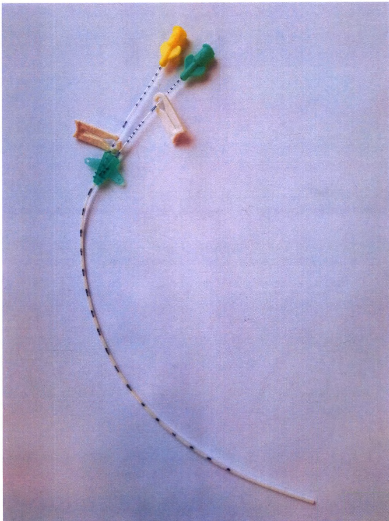
Общий вид изделия «Катетер пупочный (двухпросветный), полиуретановый (арт.1272.XX)» без предохранителя трубки катетера
