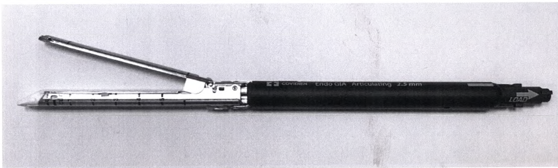
6. Одноразовый универсальный загружаемый блок изогнутой формы Endo GIA™ Auto Suture™ 60 мм - 2,5 мм;
