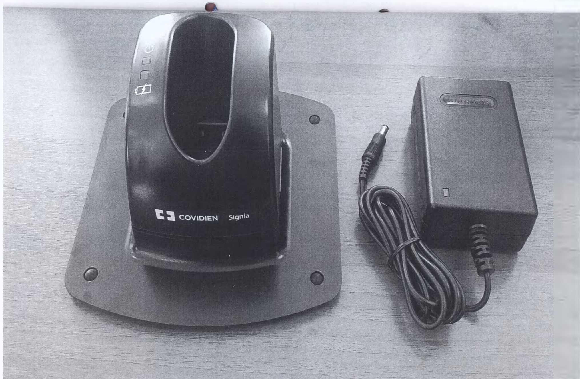
Фото 11. Зарядное устройство на одну ячейку
