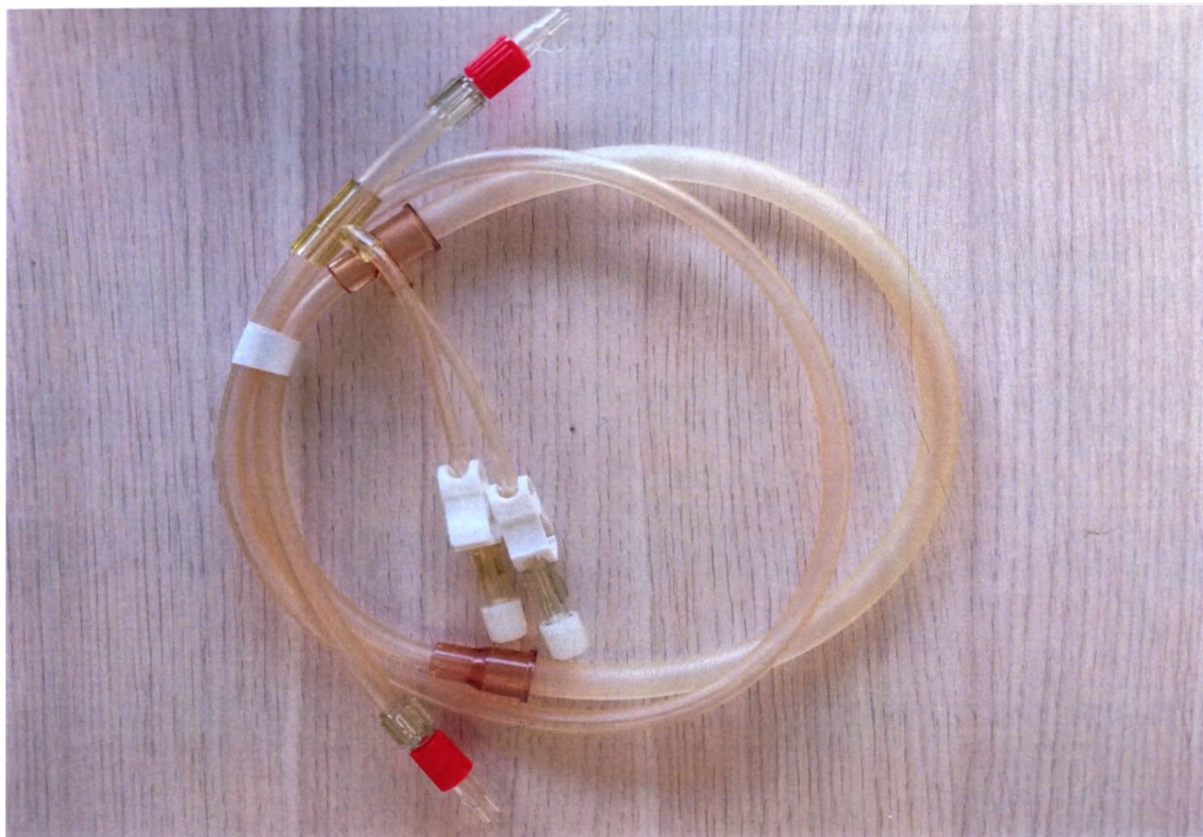
Рисунок 3 – Общий вид магистрали кровопроводящей Dialife®, модель HD-BR 003
