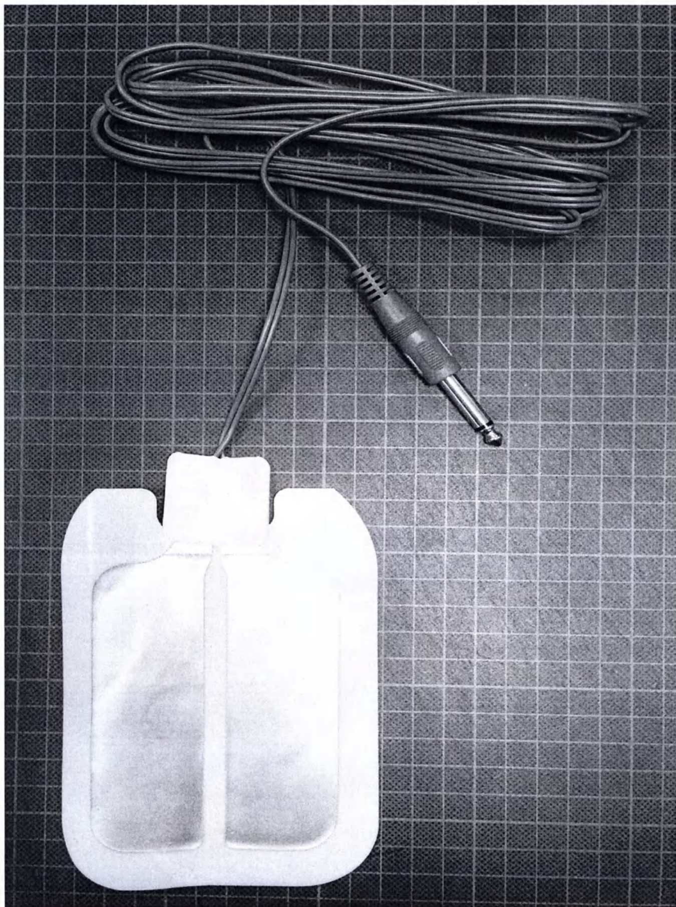
Пассивный электрод для электрохирургии с кабелем нестерильный одноразовый педиатрический двойной 2600-С/00
