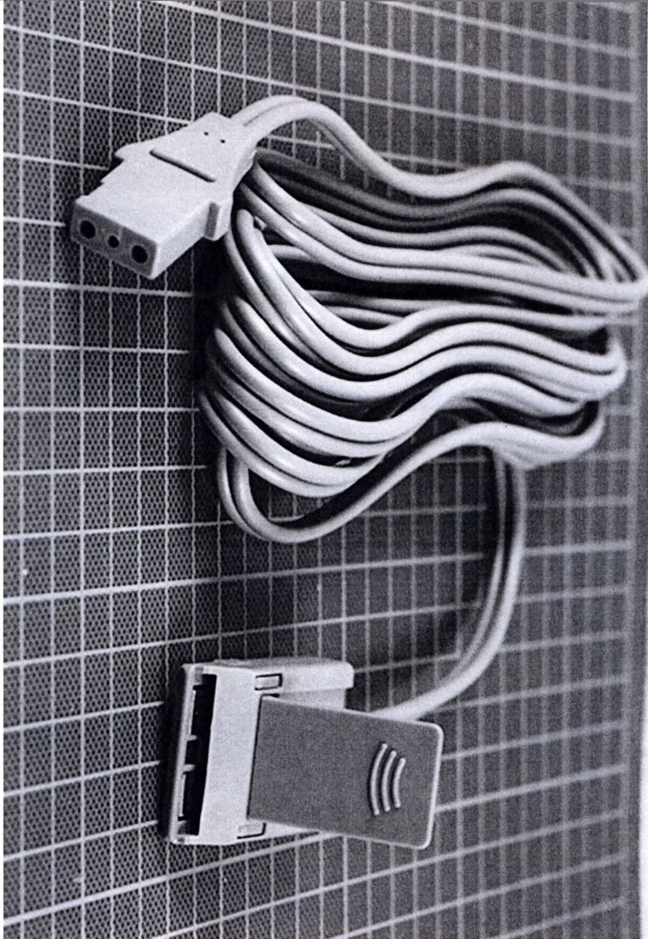
Кабель к пассивным электродам (нестерильные, многожильные) 4210 и 4210-5 (отличаются длиной)
