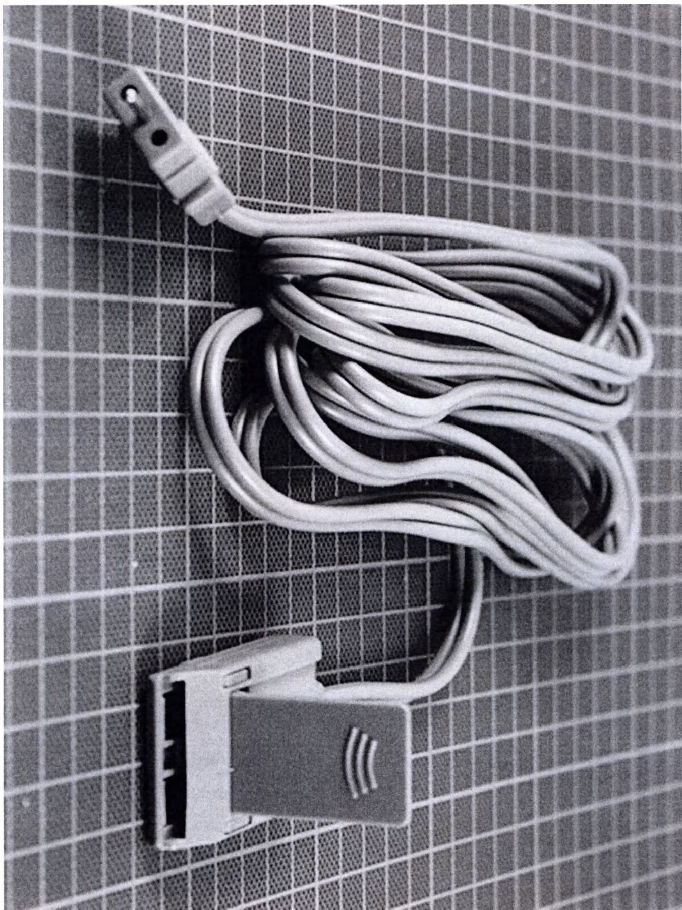
Кабель к пассивным электродам (нестерильные, многоразовые) 4212 и 4212-5 (отличаются длиной)
