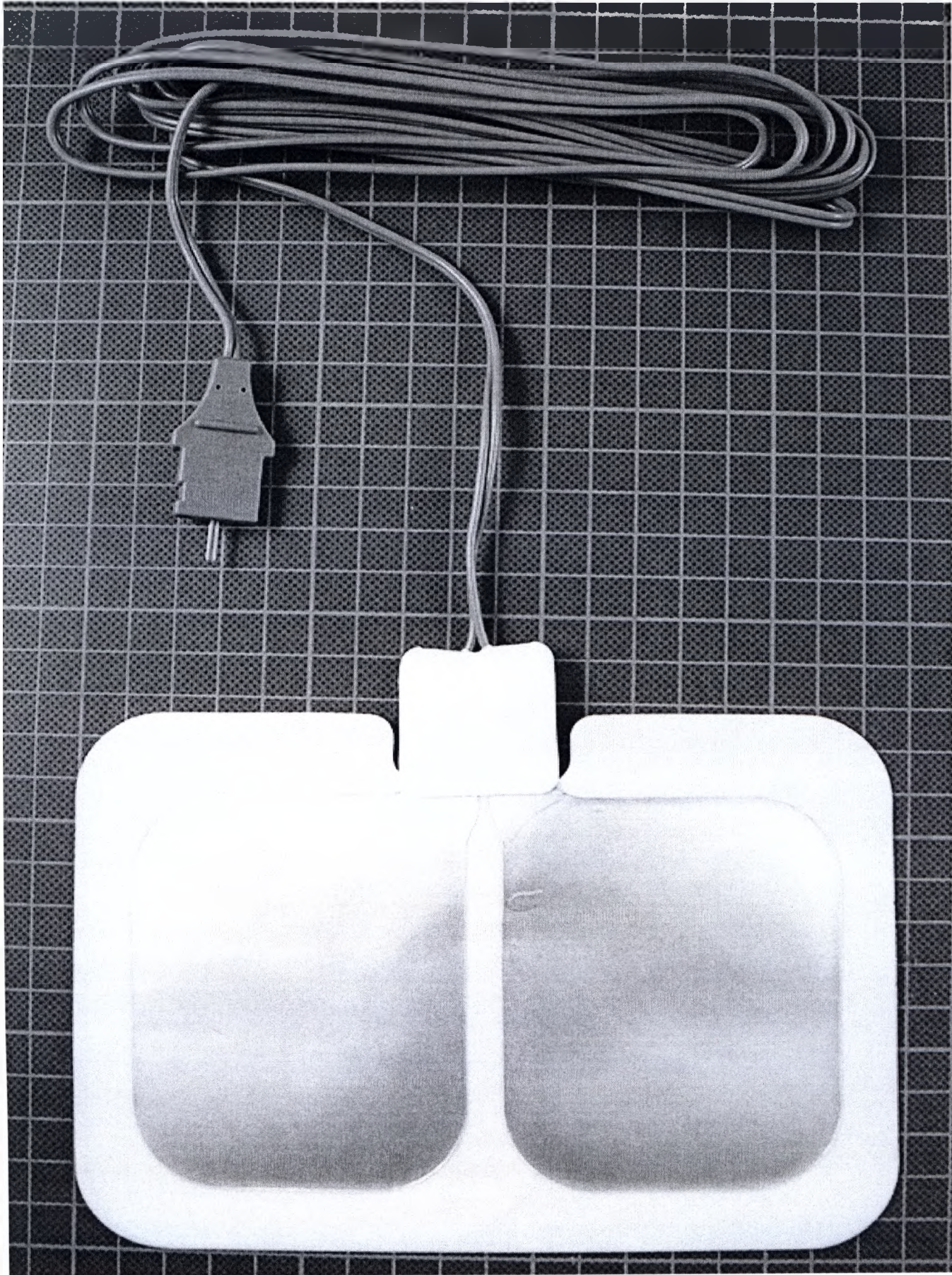
Пассивный электрод для электрохирургии с кабелем нестерильный одноразовый взрослый продолговатый двойной 2510-С/12
