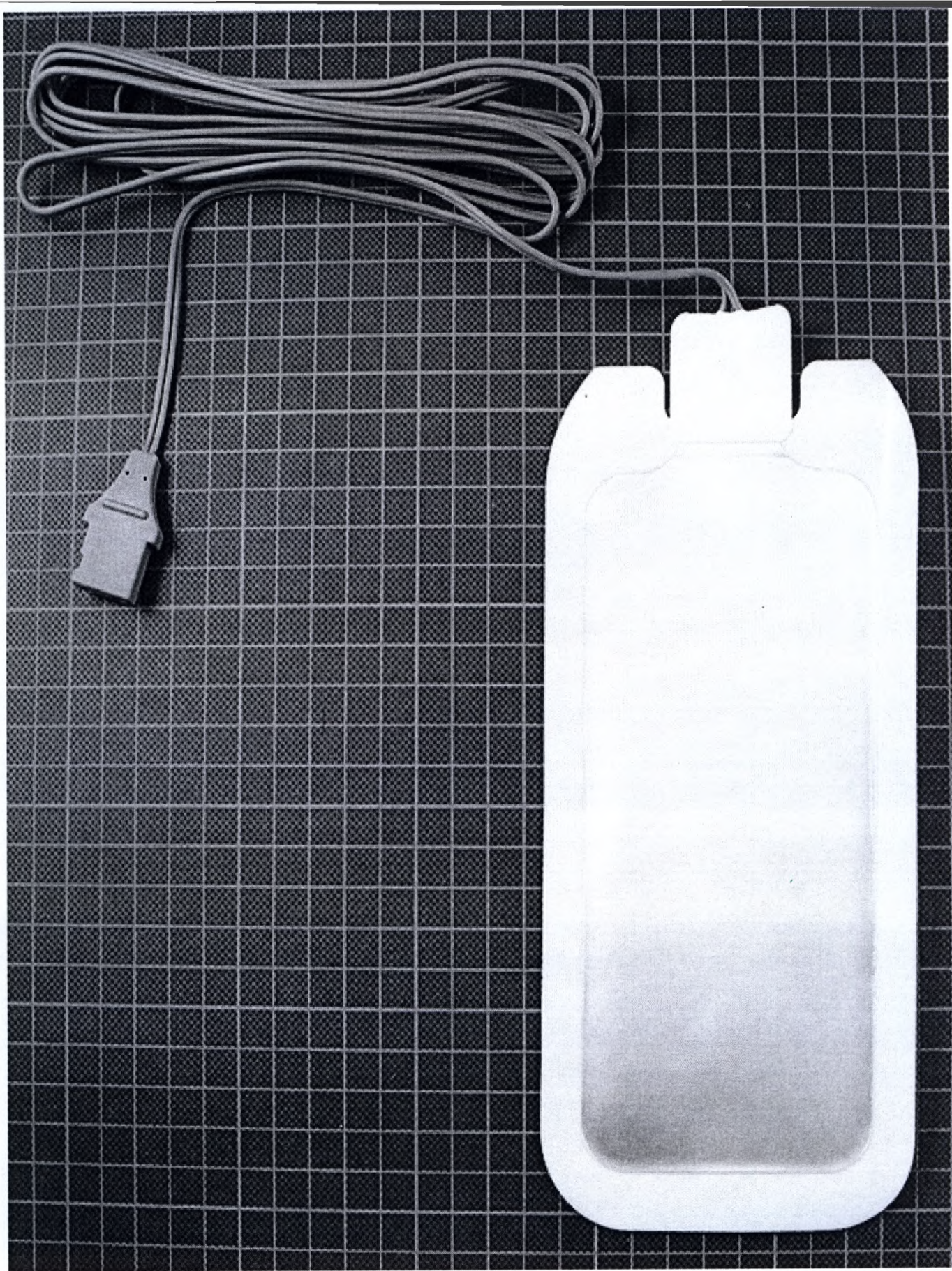
Пассивный электрод для электрохирургии с кабелем нестерильный одноразовый взрослый униполярный 2125-C/10
