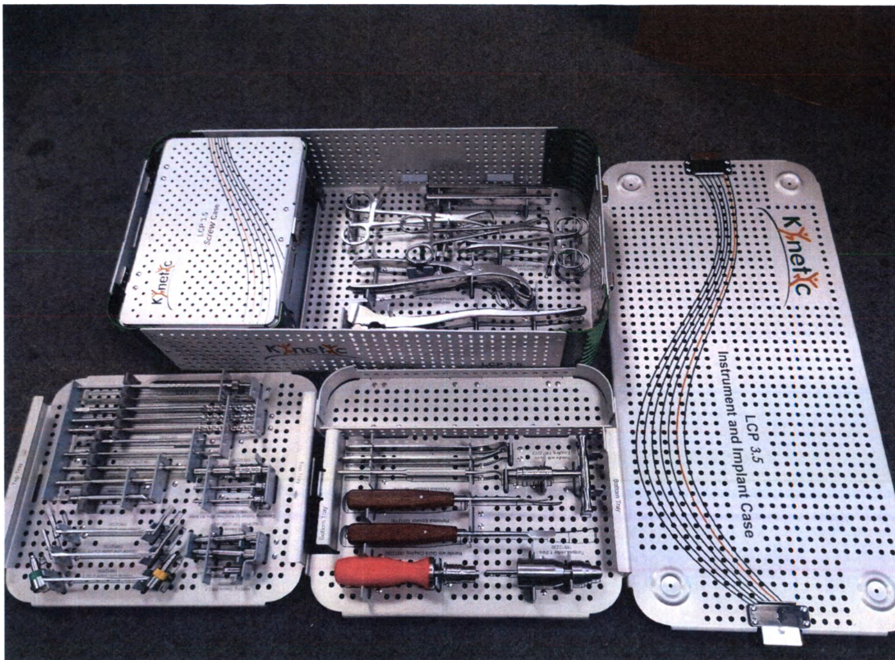
Внешний вид набора инструментов LCP3.5
