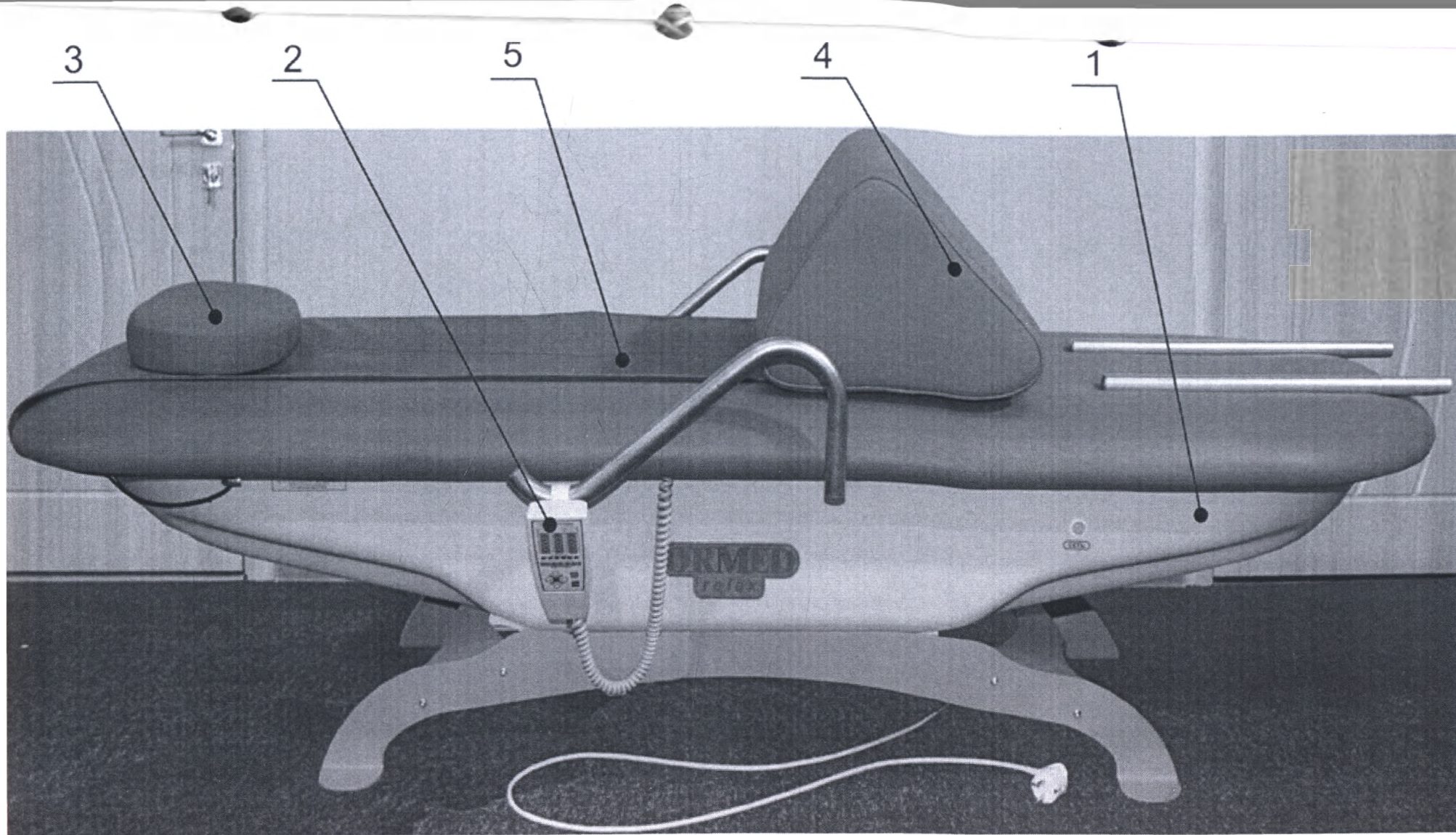
1– Установка механотерапевтическая «ОРМЕД-релакс»; 2– Пульт управления; 3– Подголовник; 4– Подколенник; 5– Накидка кушетки.
