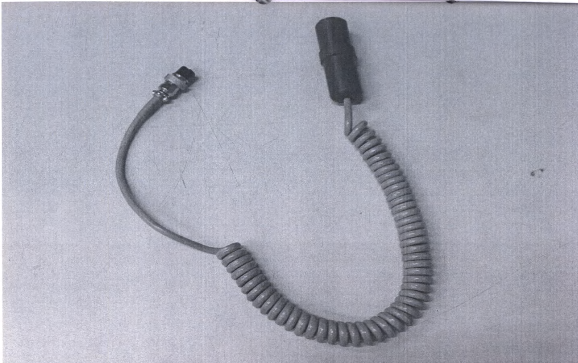
Фото 7. Общий вид составных частей медицинского изделия Установки механотерапевтические «ОРМЕД» по ТУ 32.50.50-001-22636951-2018 модели: «ОРМЕД-профессионал», «ОРМЕД-профилактик», «ОРМЕД-релакс», «ОРМЕД-тракцион», «ОРМЕД-кинезо», варианты исполнения, модели: «ОРМЕД-профессионал», «ОРМЕД-тракцион»: Кнопка пациента
