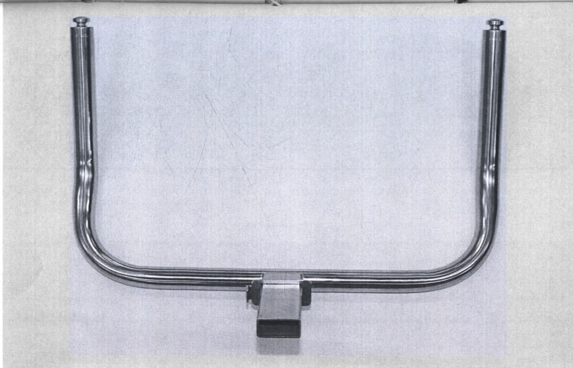
Фото 23. Общий вид составных частей медицинского изделия Установки механотерапевтические «ОРМЕД» по ТУ 32.50.50-001-22636951-2018 модели: «ОРМЕД-профессионал», «ОРМЕД-профилактик», «ОРМЕД-релакс», «ОРМЕД-тракцион», «ОРМЕД-кинезо», варианты исполнения, модели: «ОРМЕД-тракцион»: Рычаг вытяжения
