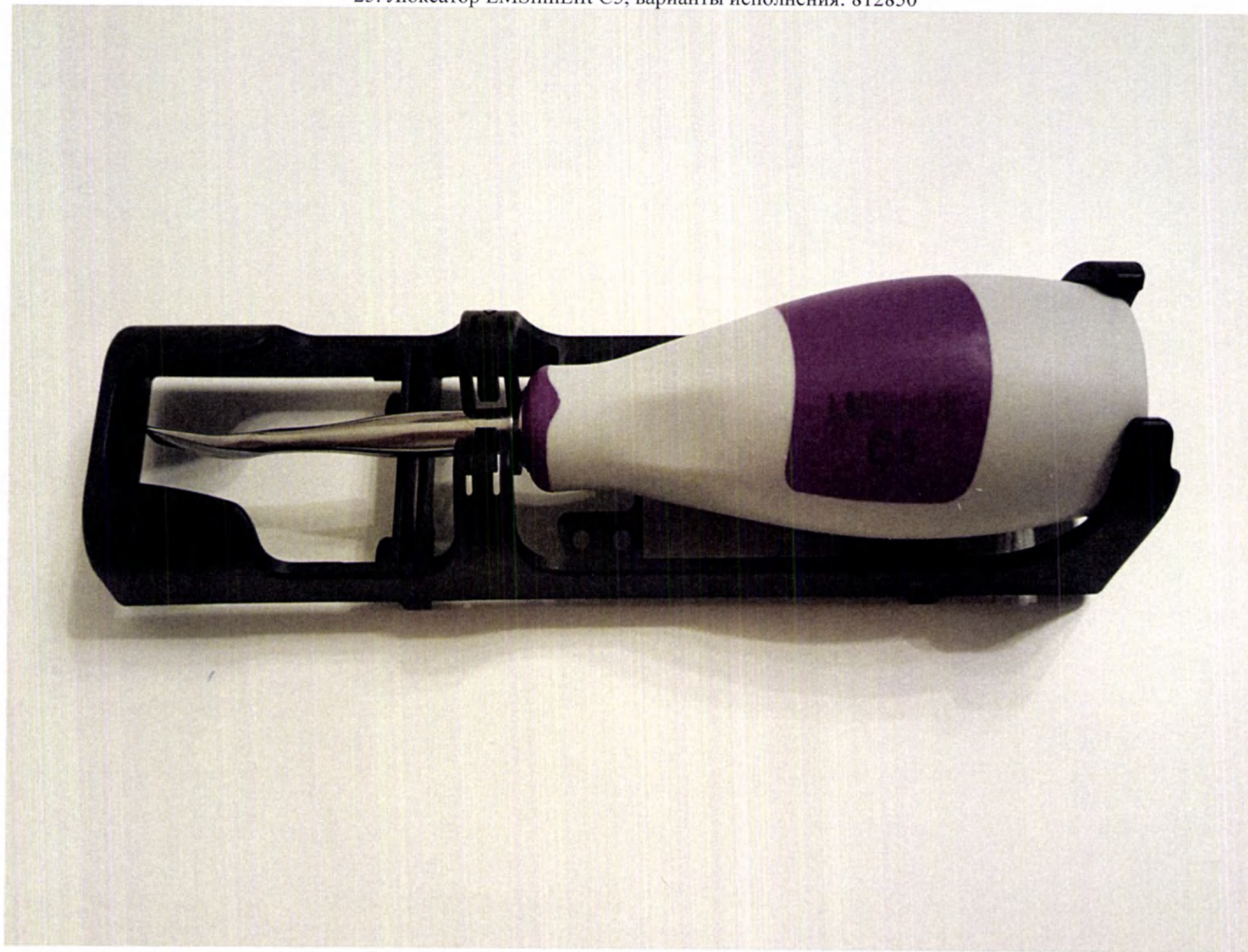
25. Люксатор LMSlimLift C5, варианты исполнения: 812850
