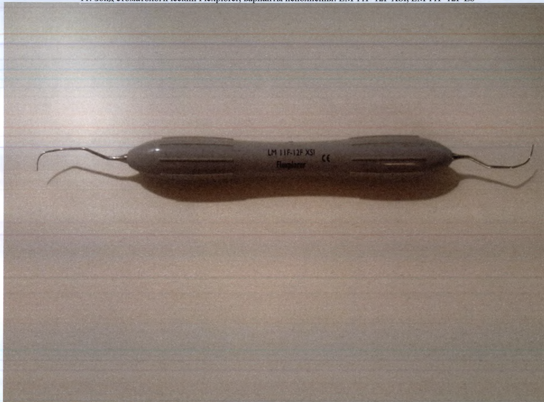
11. Зонд стоматологический Flexplorer, варианты исполнения: LM 11F-12F XSI, LM 11F-12F ES
