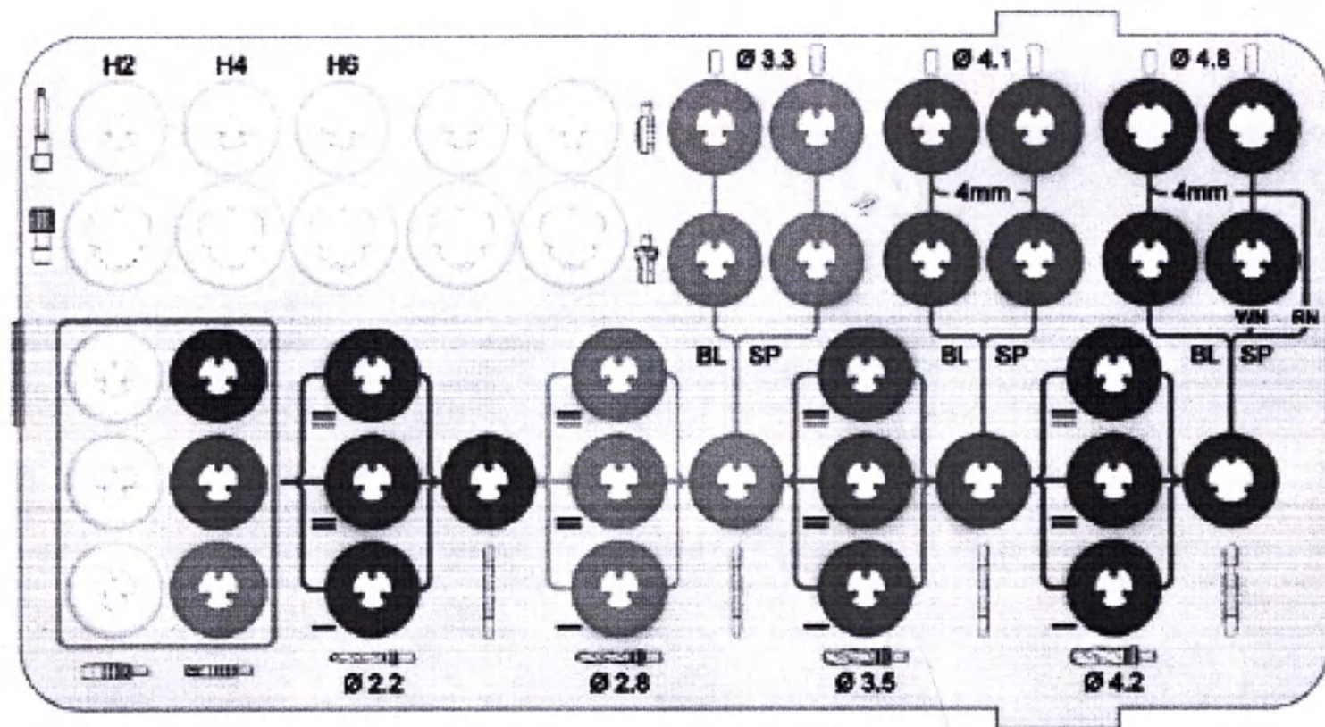
Фото 48 — Лоток для инструментов стоматологических для установки дентальных имплантатов BL, TL для направленной хирургии для модуля В
