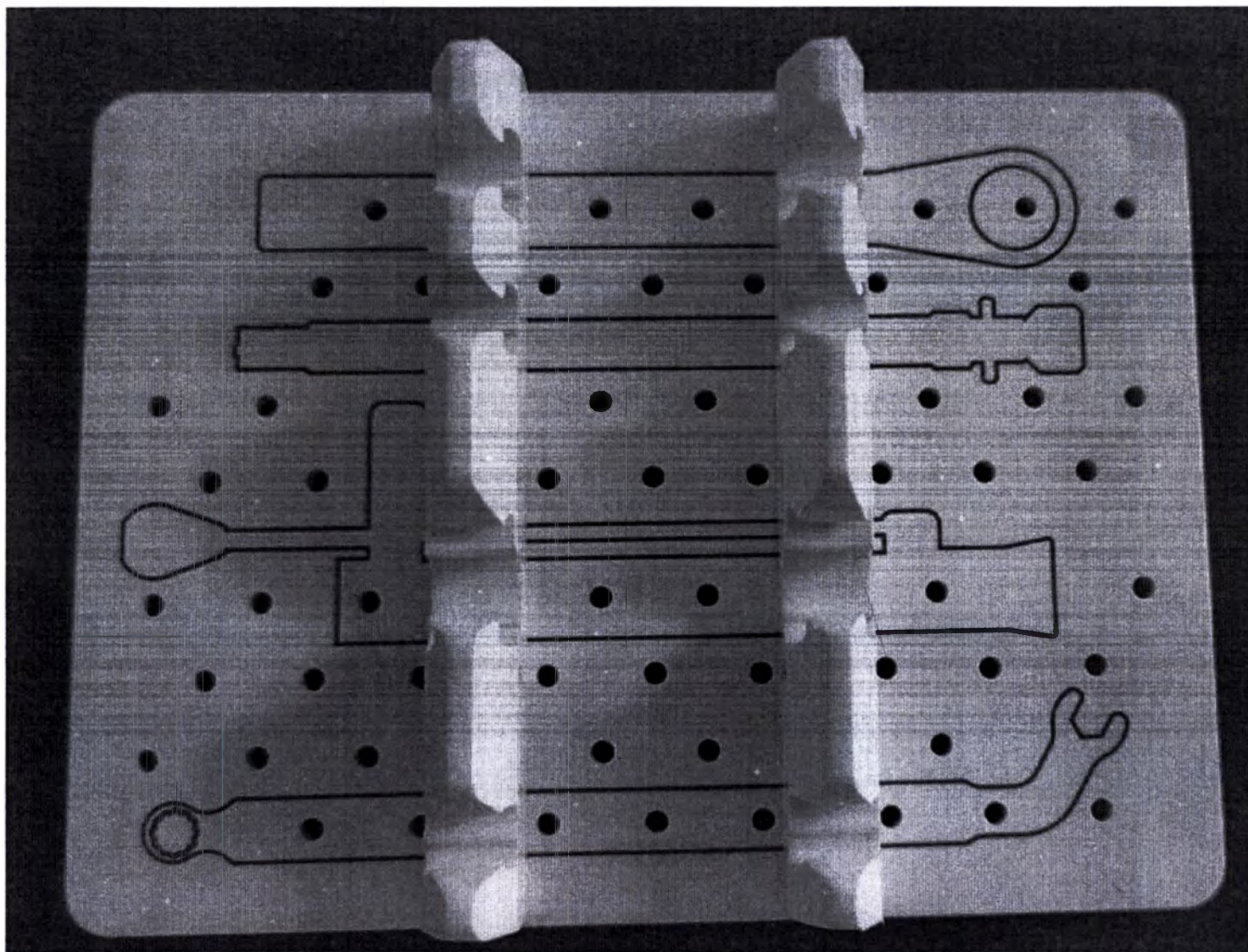
Фото 14 – Лоток для ключа реверсивного для модуля А
