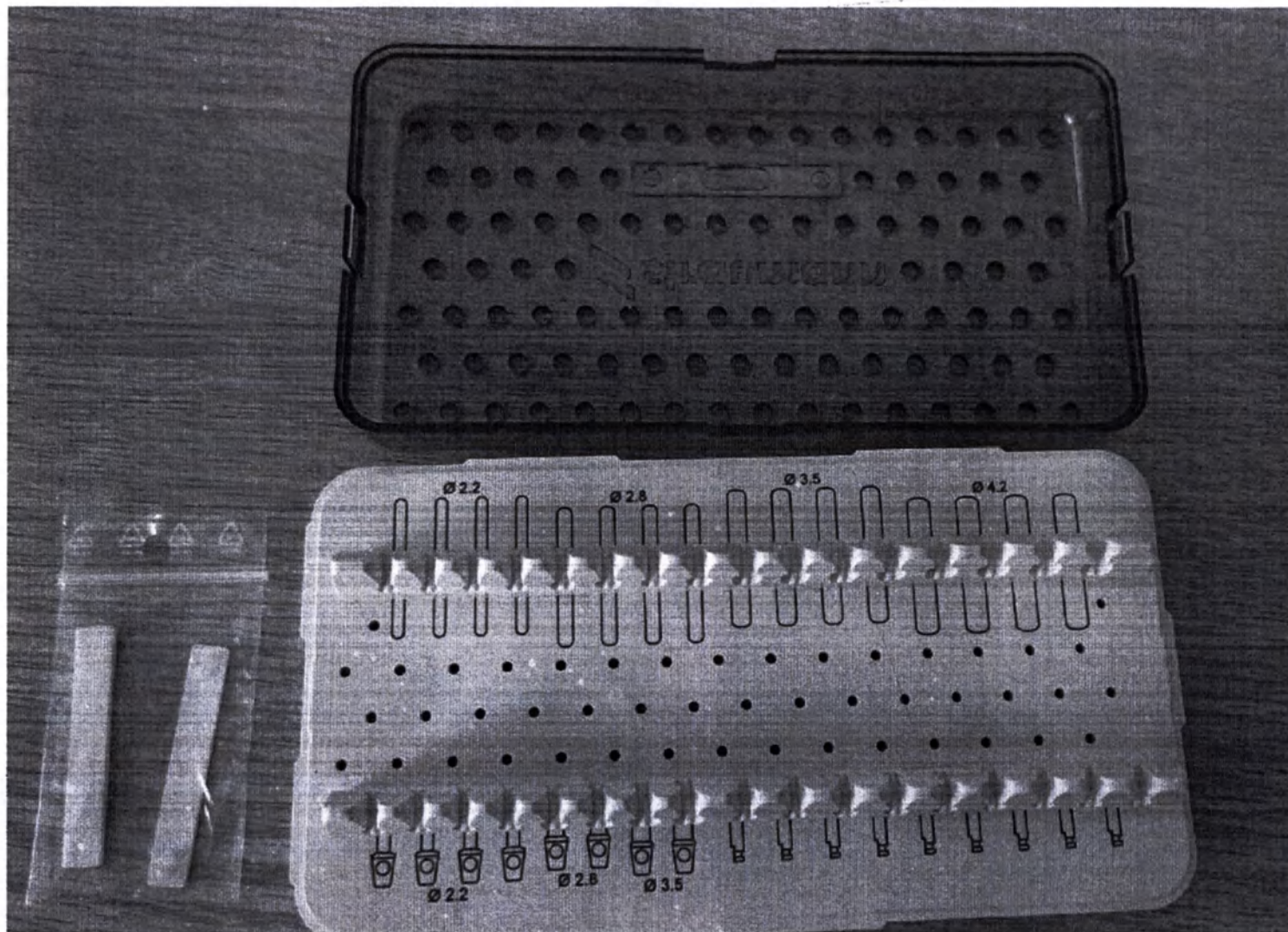
Фото 59 — Кассета модульная Straumann для инструментов стоматологических вспомогательных, модуль С; с Пластинами для этикеток в первичной упаковке
