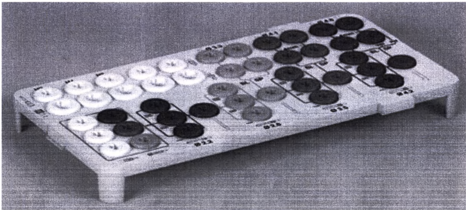
Фото 49 — Лоток для инструментов стоматологических для установки дентальных имплантатов BL, TL для направленной хирургии для модуля В
