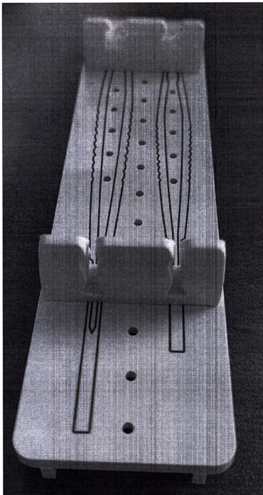
Фото 27 – Лоток для пинцета для модуля А
