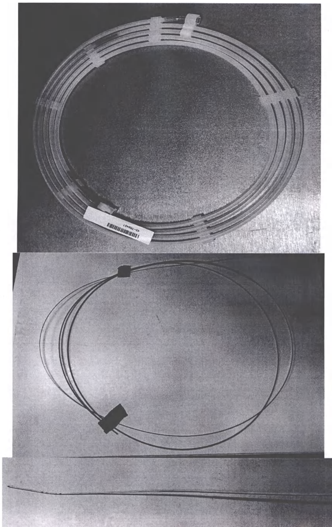
Система Azur CX 35 для спиральной эмболизации периферических сосудов (отсоединяемая)
