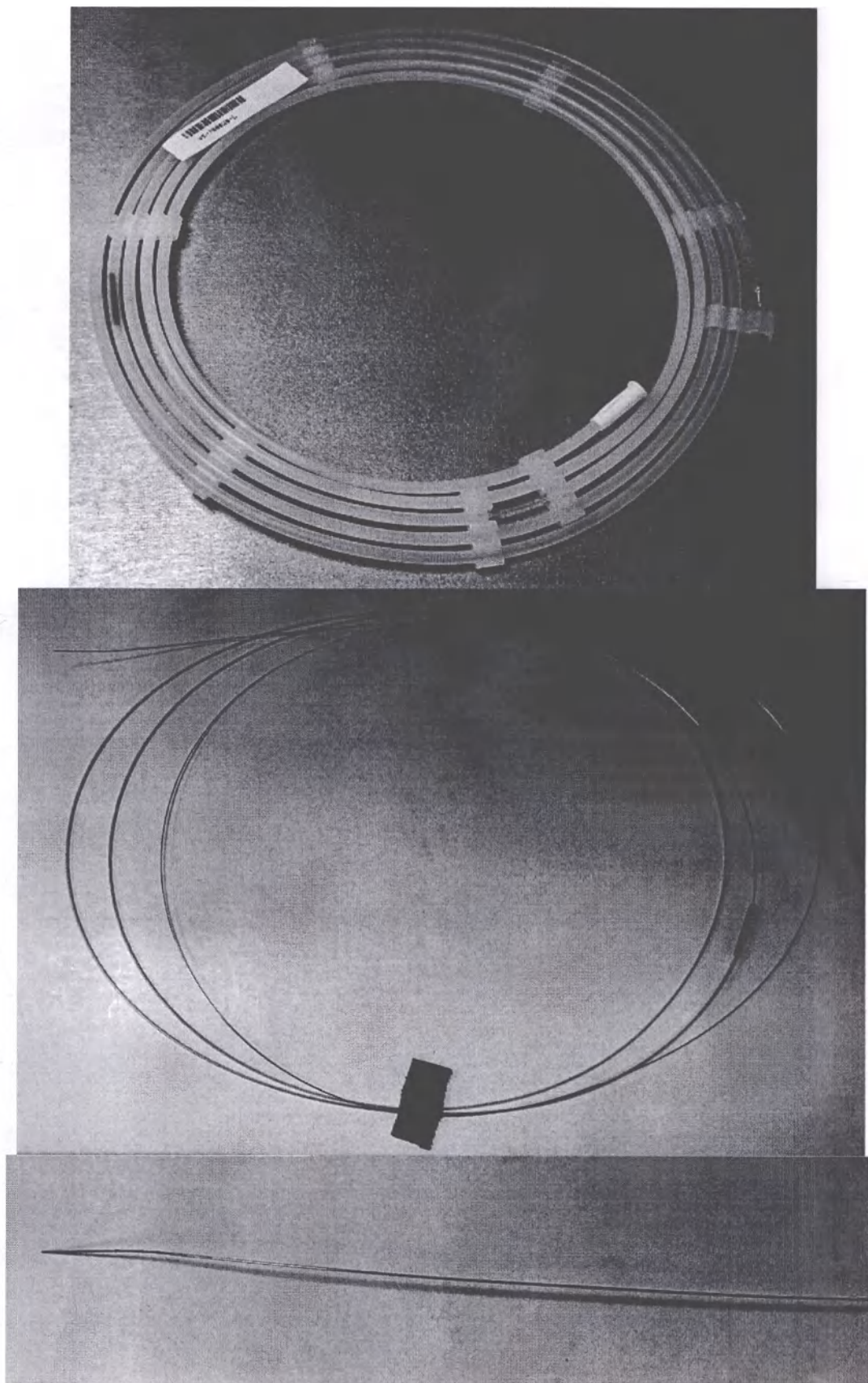
Система Azur CX 18 для спиральной эмболизации периферических сосудов (отсоединяемая)
