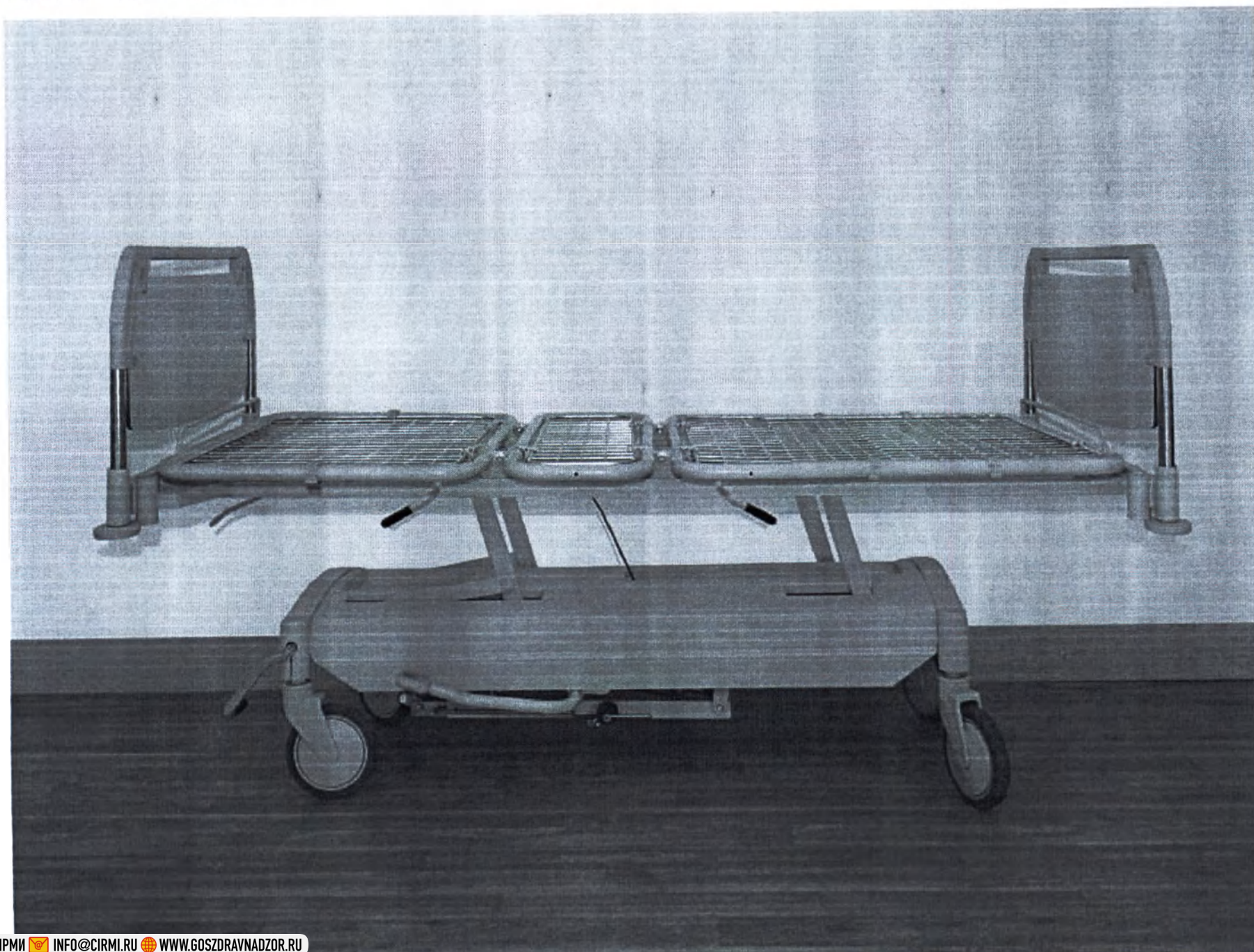
Фото 3.8. Модель К-ДЗМО-2-3-Г.
