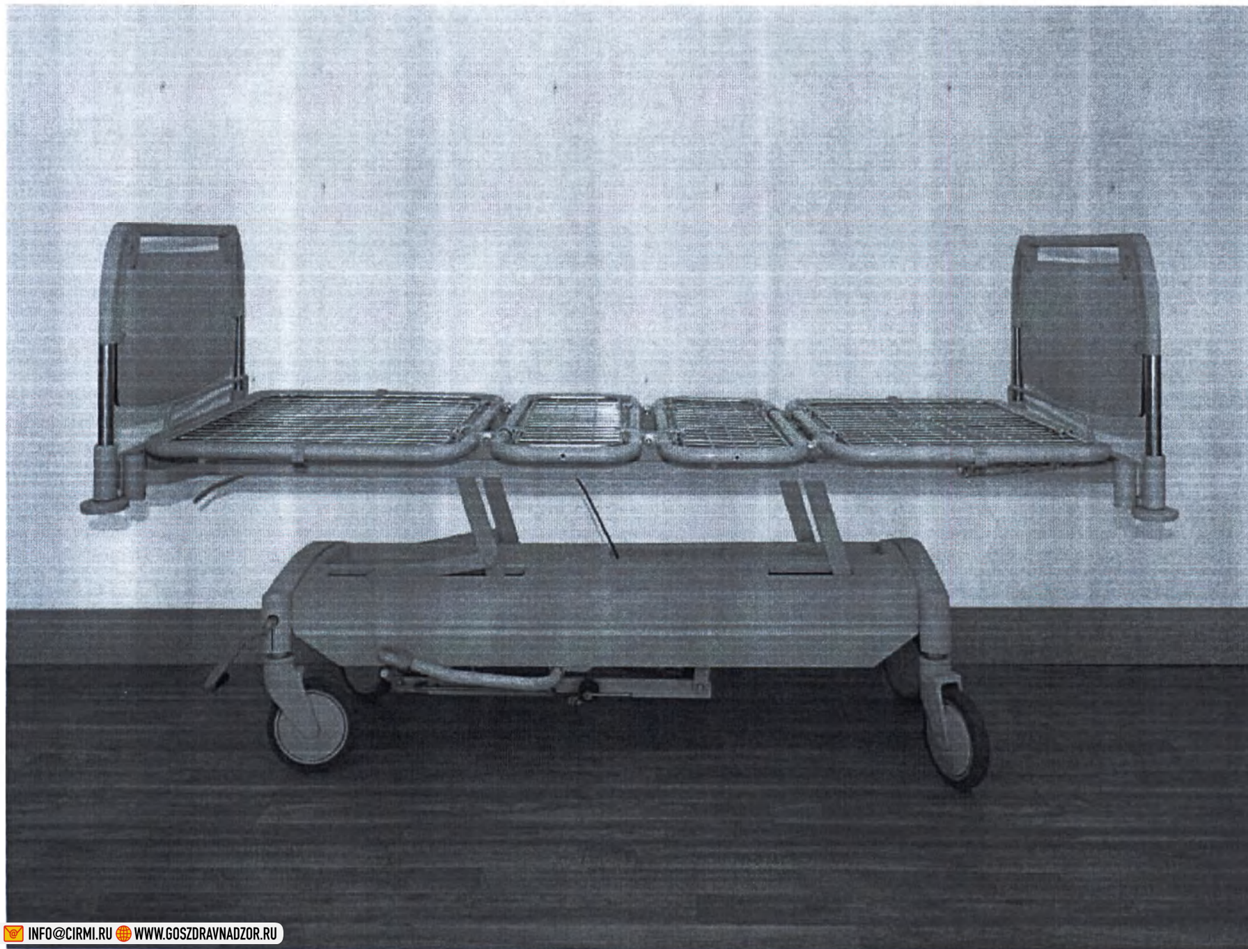
Фото 4.7. Модель К-ДЗМО-2-4-Р.
