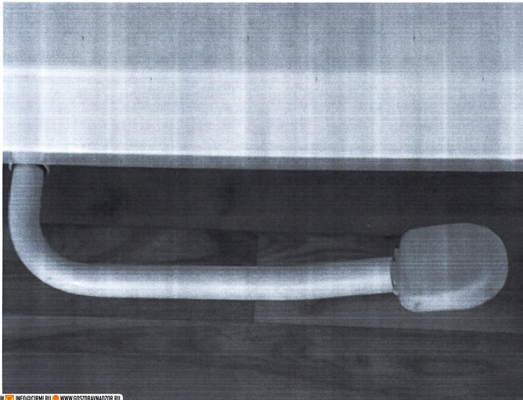
Фото 5.18. Педаль управления выдвижным пятым колесом.
