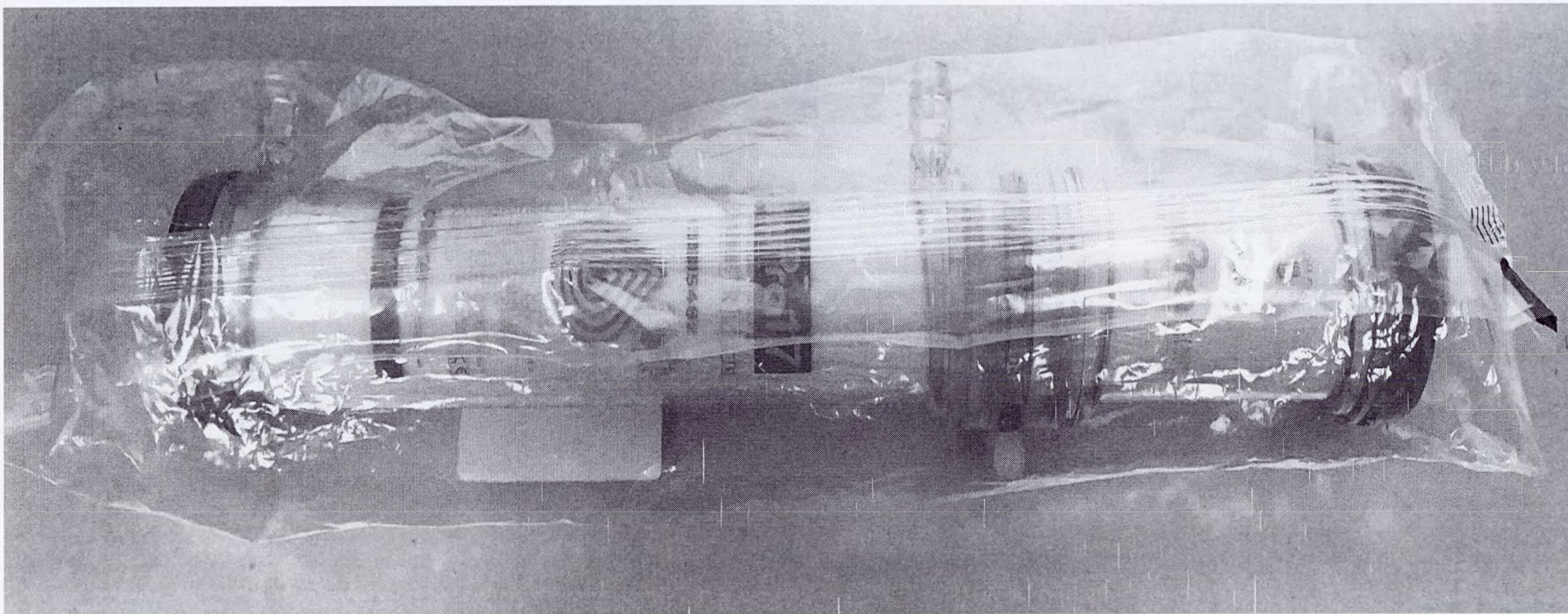
Капиллярный диализатор – SUPRA 17
