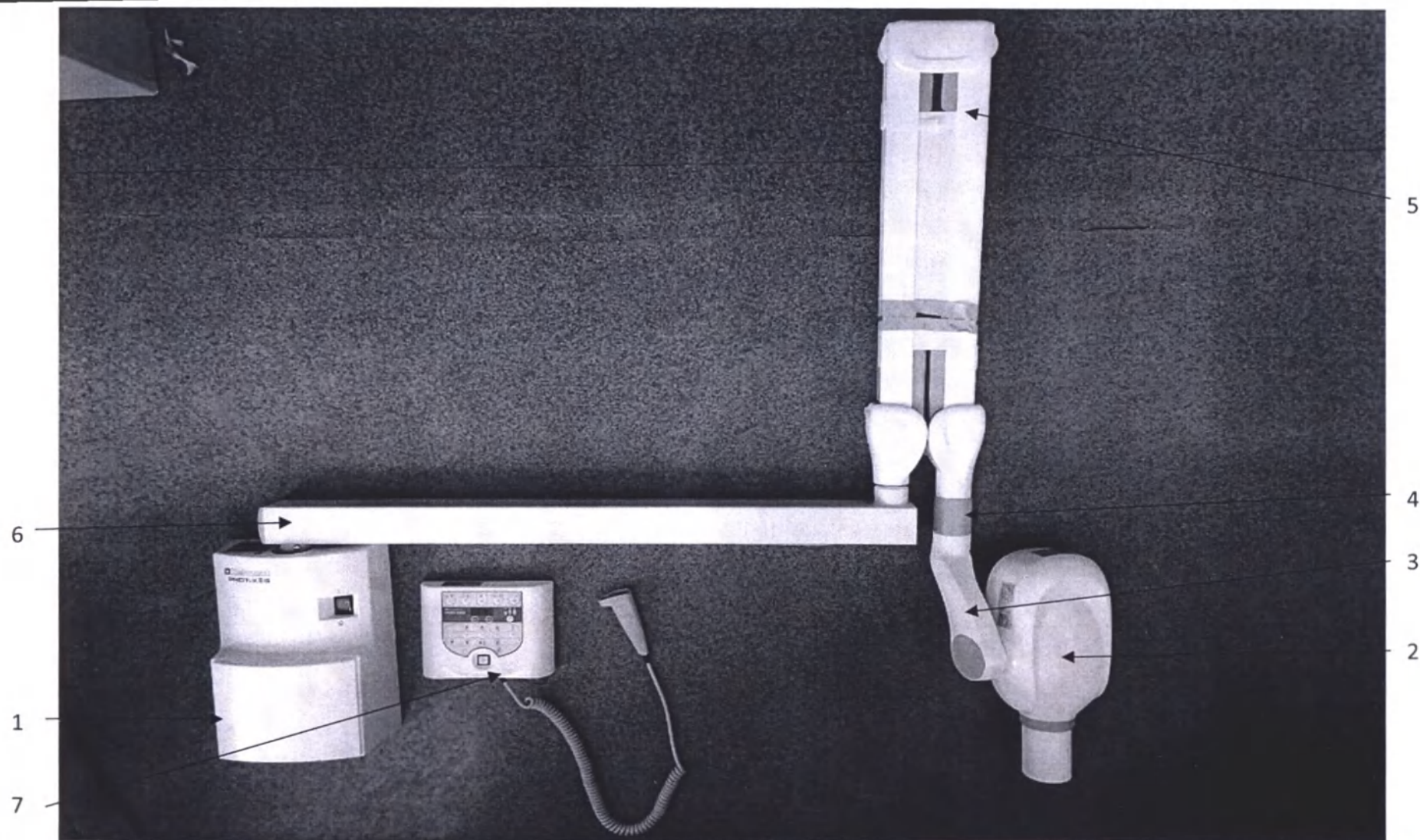
Установка PHOT-X IIs 505, тип WK (внешний вид установки PHOT-X IIs 505LCD, тип WK идентичен, кроме вспомогательного контроллера): 1 – главный контроллер, 2 – тубус рентгеновской трубки, 3 – хомут, 4 – манжета рычага, 5 – балансировочный шарнирный рычаг, 6 – горизонтальный рычаг, 7 – контроллер вспомогательный с ручным выключателем
