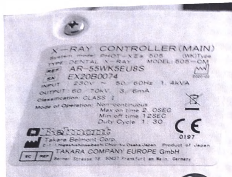
Маркировка установки PHOT-X IIs 505, тип WK
