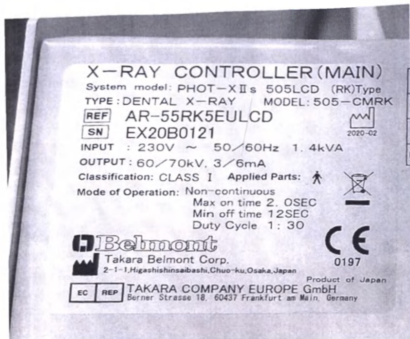
Маркировка установки PHOT-X IIs 505LCD, тип RK
