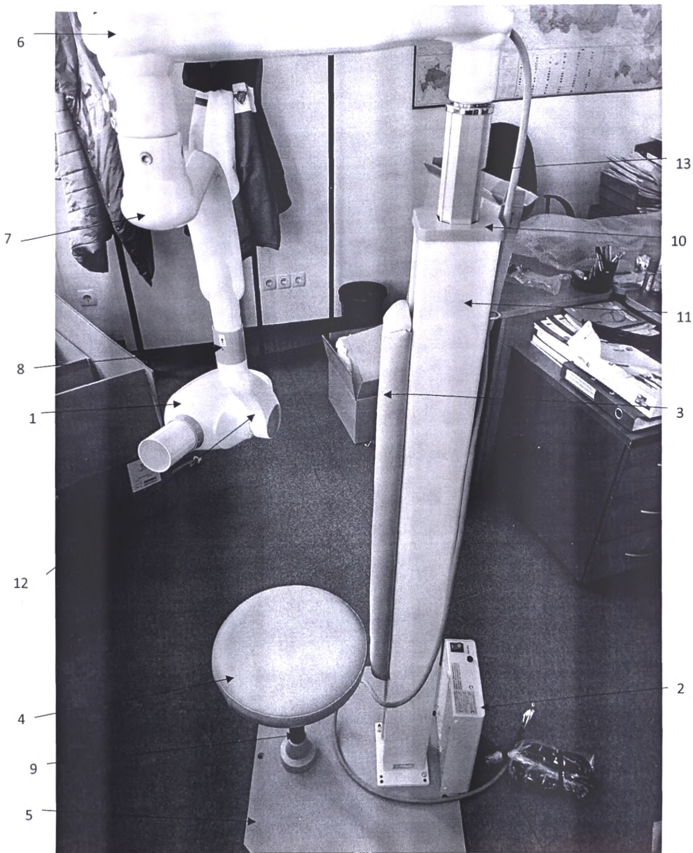
Установка PHOT-X IIs 505LCD, тип RK (внешний вид установки PHOT-X IIs 505, тип RK идентичен, кроме вспомогательного контроллера): 1 – тубус рентгеновской трубки, 2 – главный контроллер, 3 – подушка спинки, 4 – сиденье, 5 – плита основания, 6 – шарнирный рычаг прямой, 7 – шарнирный рычаг изогнутый, 8 – манжета рычага, 9 – газлифт, 10 – крышка колонны, 11 – колонна, 12 – хомут, 13 – скользящая опора
