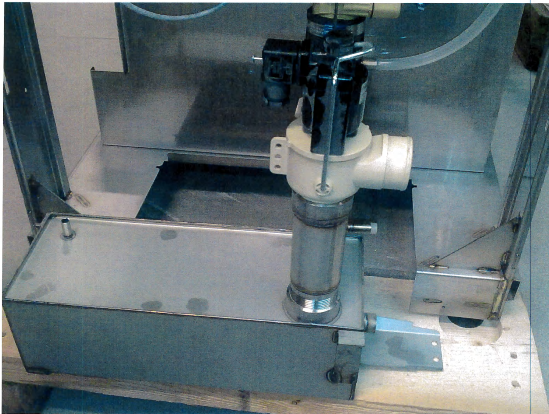
23. Конденсатор влаги
