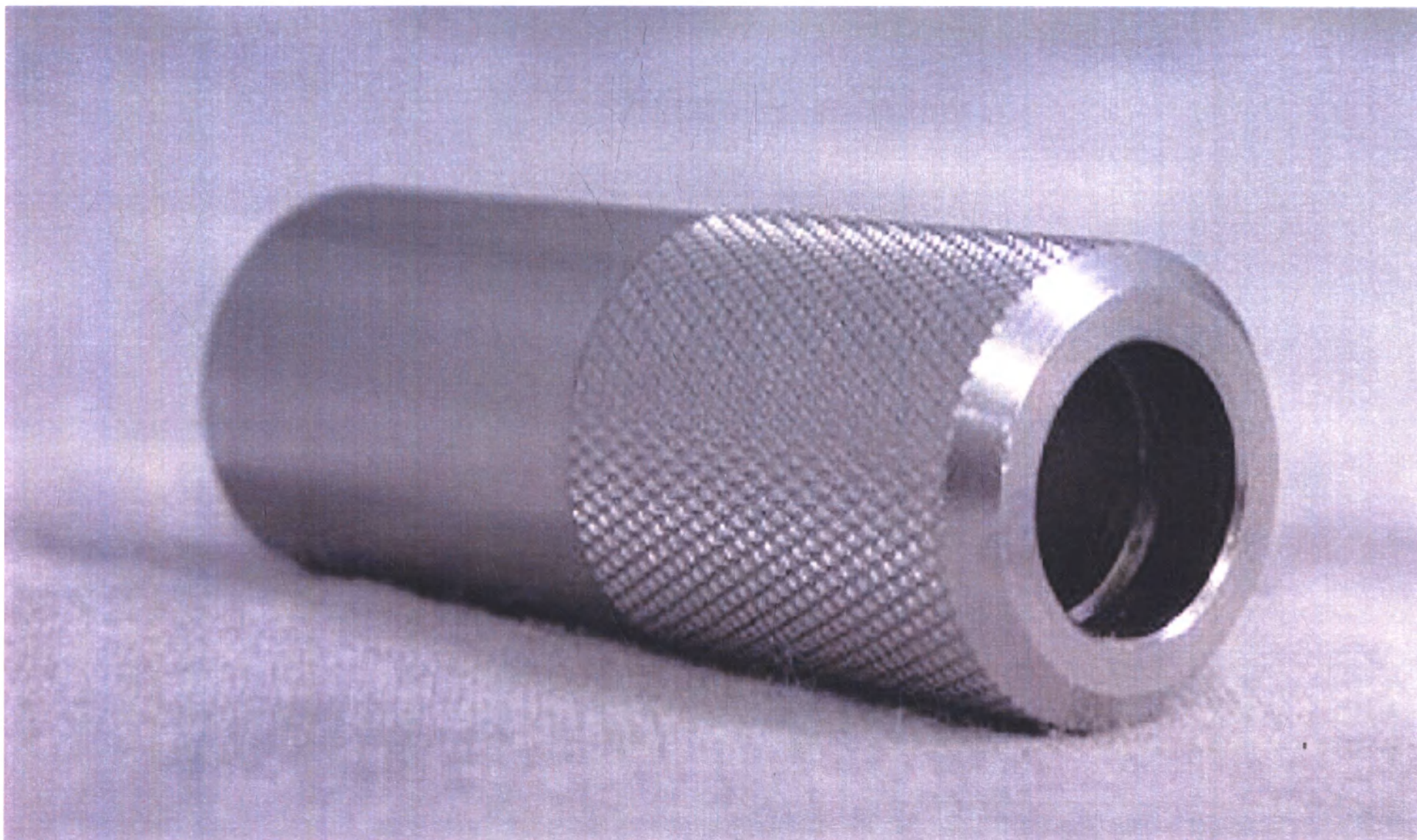
Адаптер Safelight к оптике Wolf.
