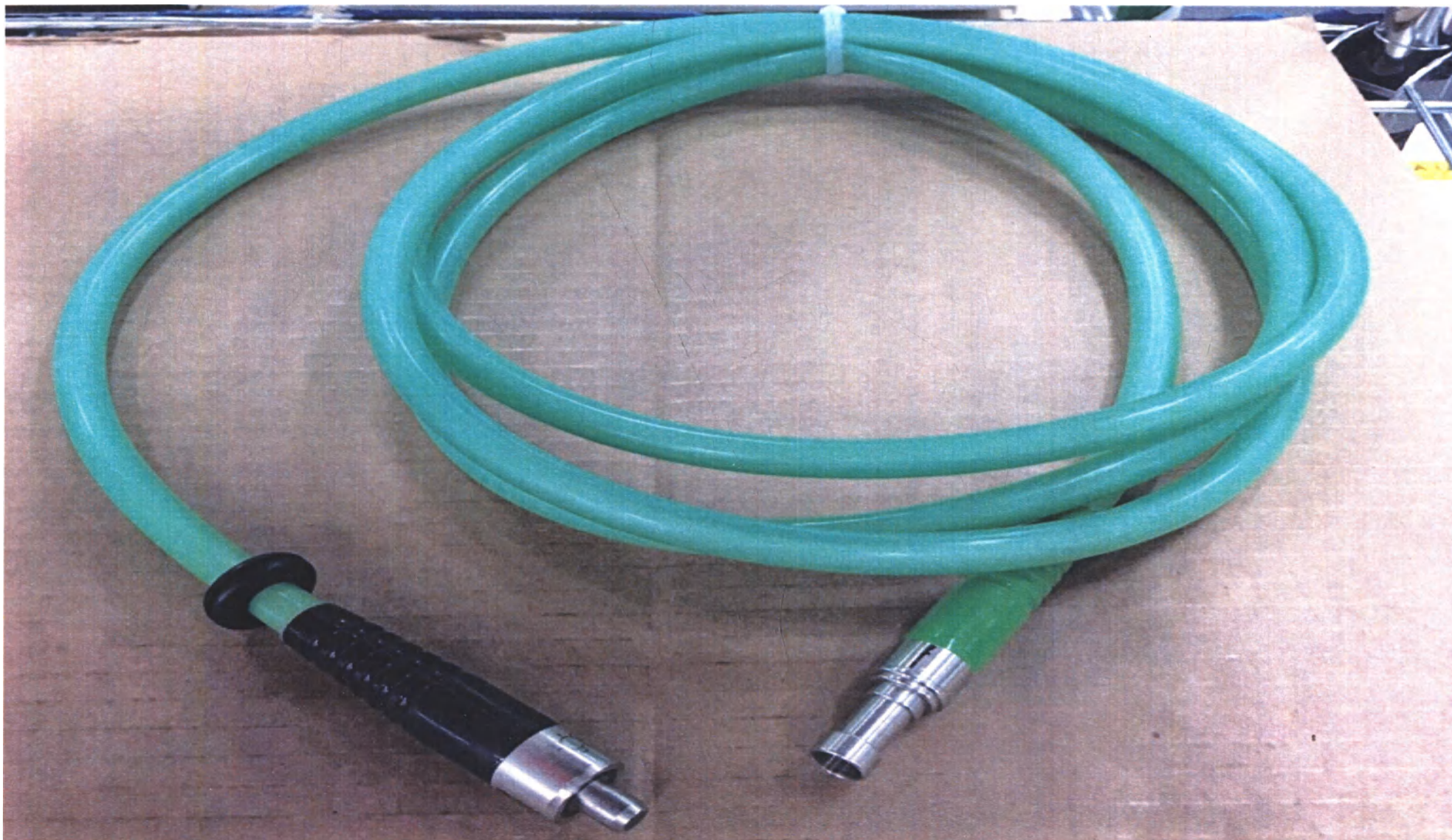
Кабель световодный фиброоптический AIM SafeLight 5 мм x 3 м.
