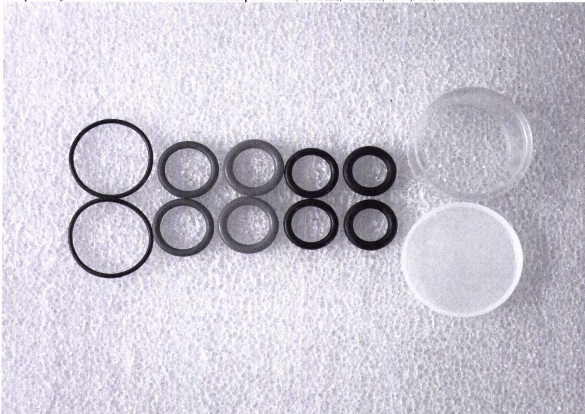
12. Набор колец уплотнительных в пластиковом контейнере:- Ø11 мм, - Ø12 мм, - Ø13 мм, - Ø14,5 мм, - Ø24 мм.
