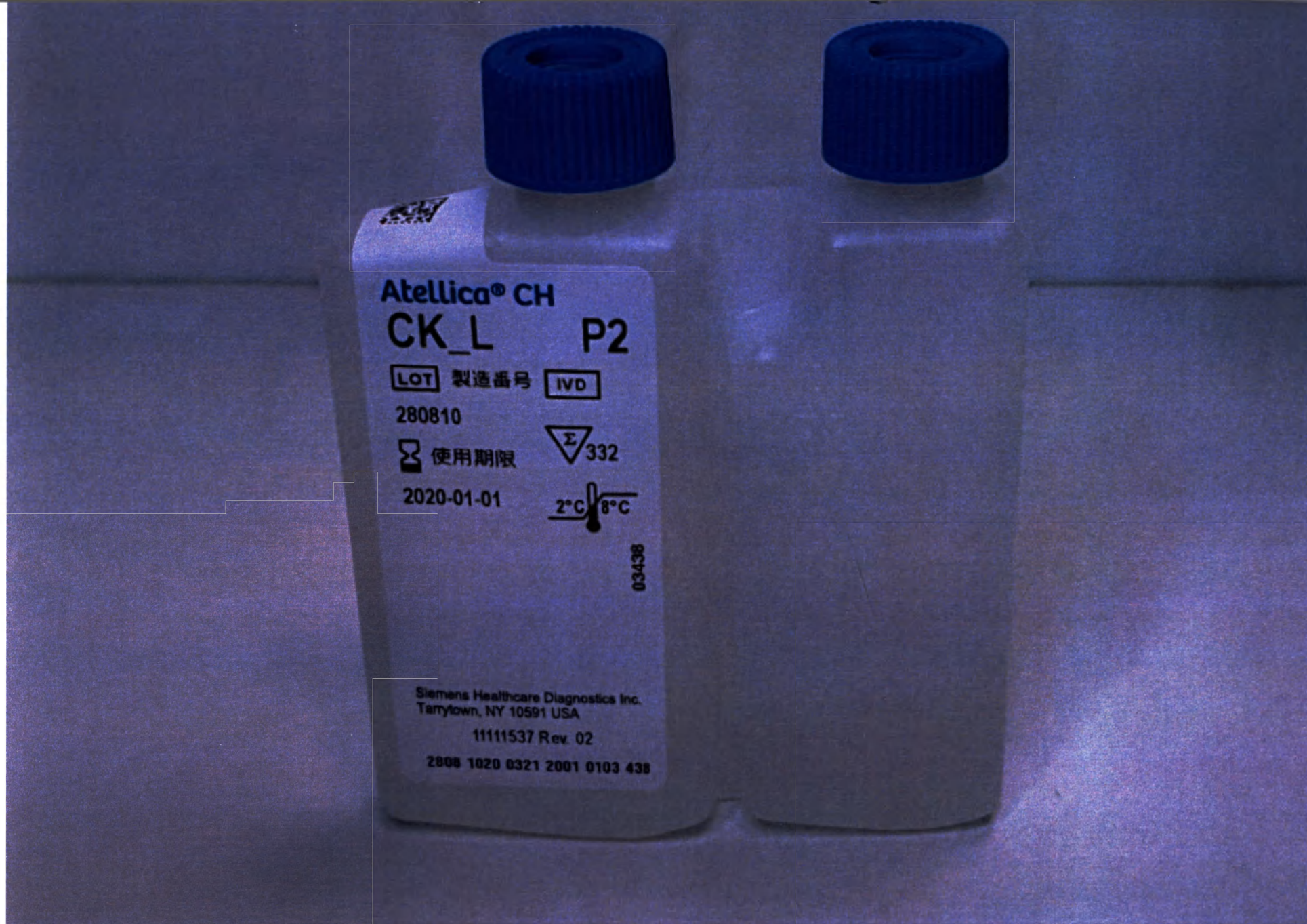
Рисунок 3 Набор реагентов для определения креатинкиназы на анализаторах биохимических серии Atellica (Atellica CH Creatine Kinase (Atellica CH CK_L)): общий вид, упаковка 2
