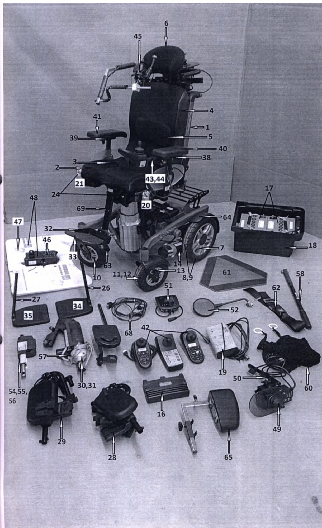
«Кресло-коляска для инвалидов «МЕYRA», с электроприводом, прогулочного и комнатного исполнения 1.616 «iChair MC S» повышенной проходимости, с принадлежностями»
