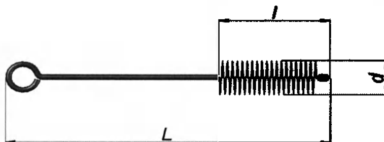
а.) Щетки с наконечником
