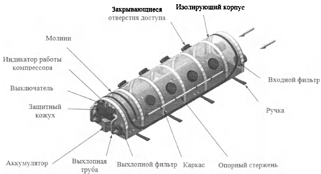
Рисунок 1 – Устройство изолятора NP-320
