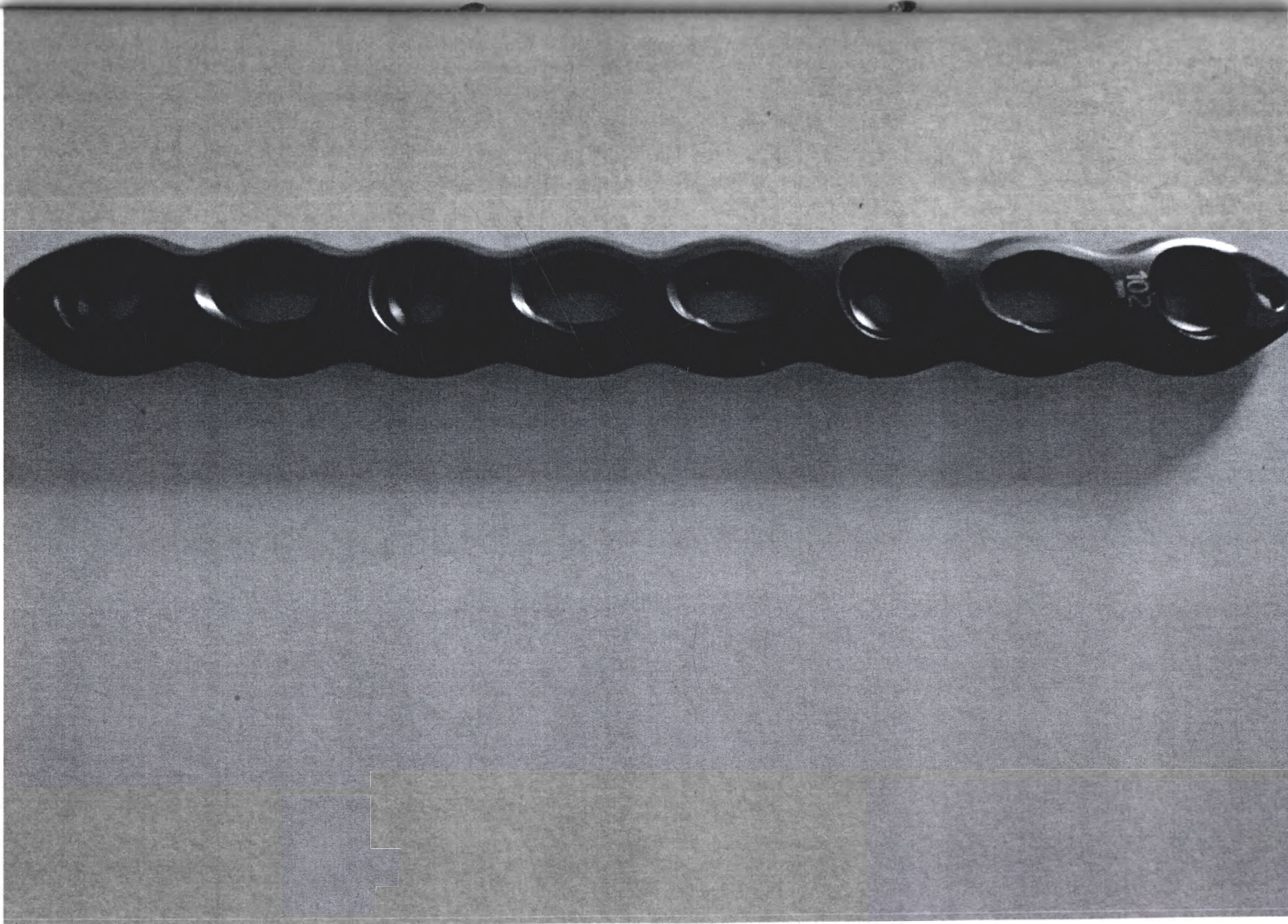
Пластина компрессионная, узкая, прямая, 3-10 отверстий.
