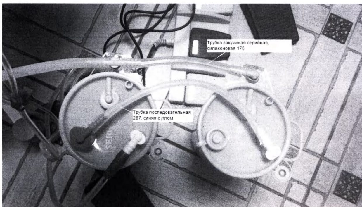
Общий вид соединения контейнеров с мешками для аспирации между собой и с вакуумным аспиратором
