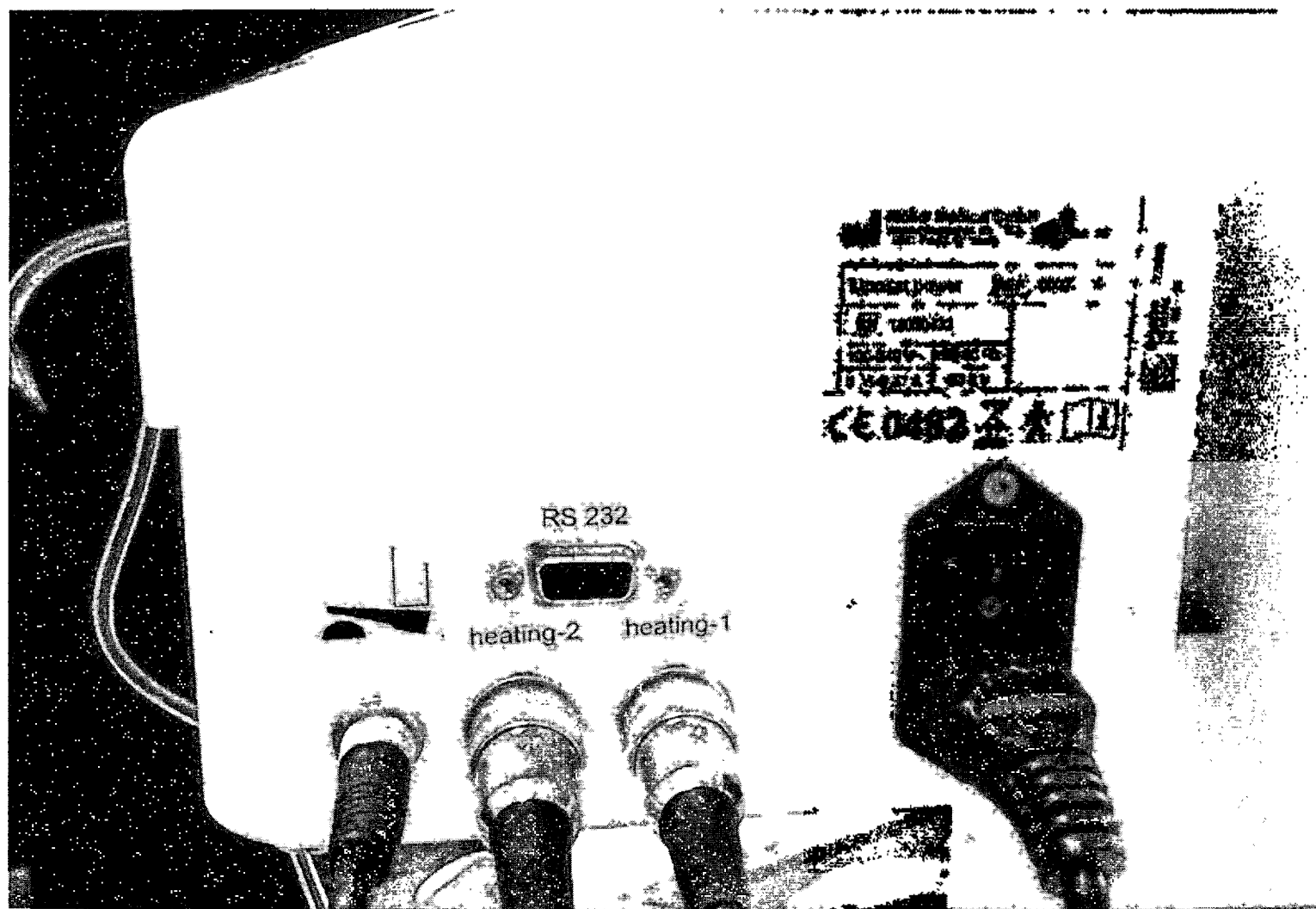
Общий вид (сбоку): Насос инфильтрационный Liposat power, артикул 00002274
