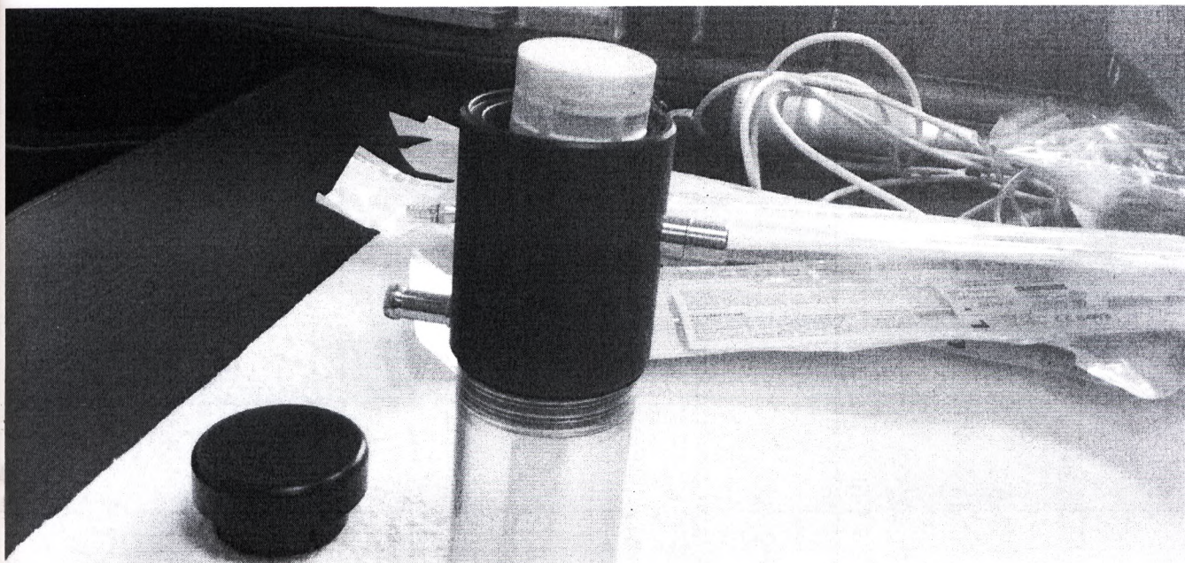
Общий вид размещения изделия «Фильтр гидрофобный для прибора (защиты от протечек), артикул 00002297» в устройстве «Защита от протечек для гидрофобного фильтра, артикул 00002299»
