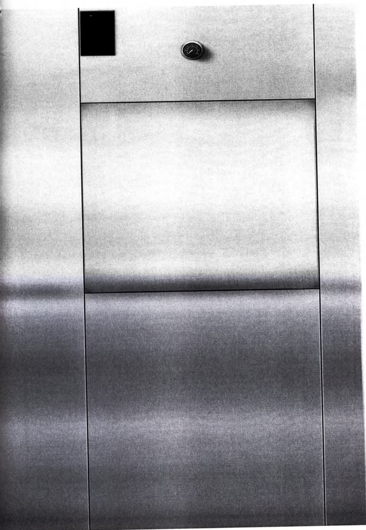
СТЕРИЛИЗАТОР ПАРОВОЙ ГОРИЗОНТАЛЬНЫЙ JSM 250L 2PD ПРОХОДНОЙ (С ДВУМЯ ДВЕРЬМИ). ВИД СЗАДИ (СТОРОНА ВЫГРУЗКИ).
