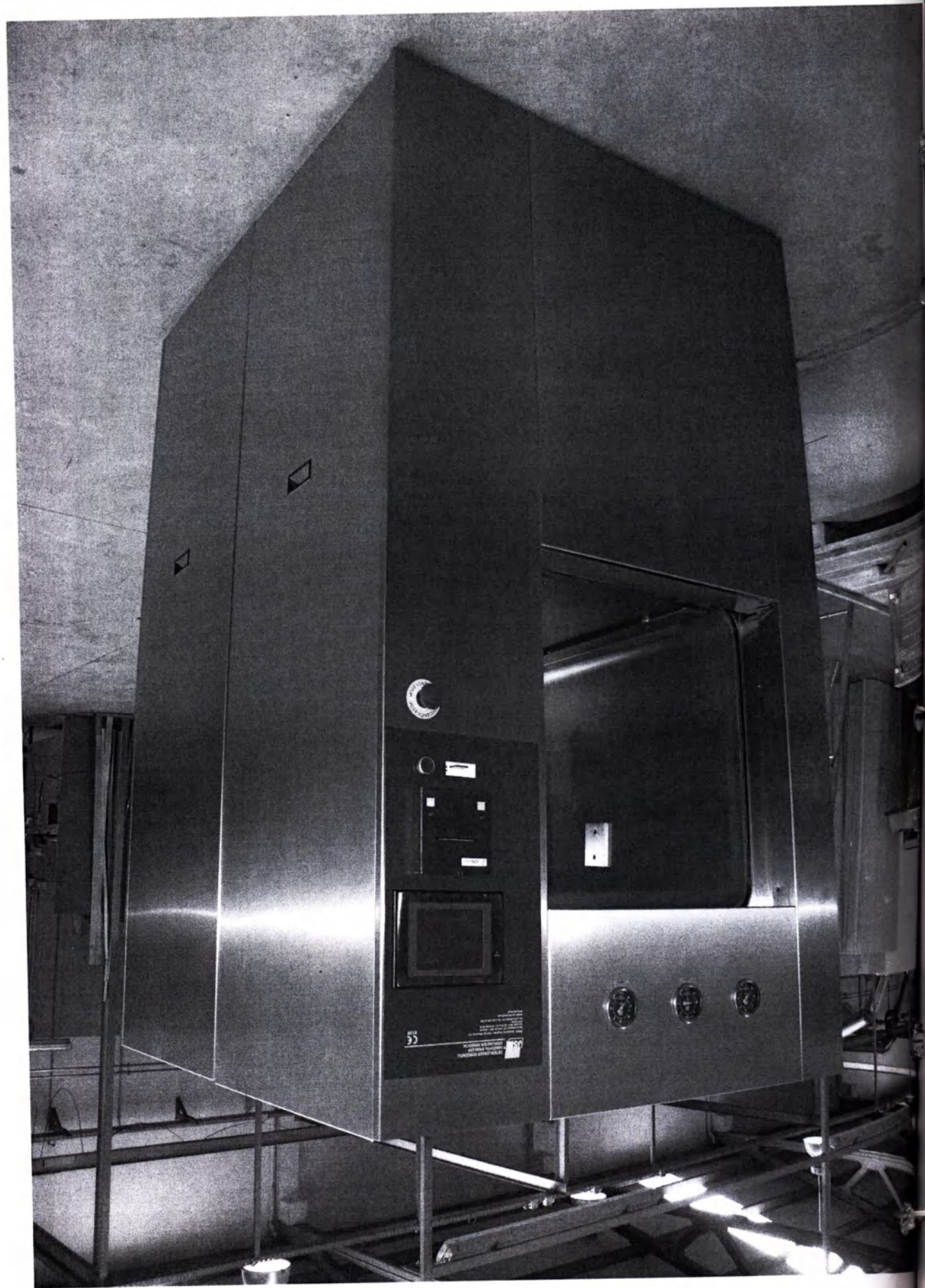
СТЕРИЛИЗАТОР ПАРОВОЙ ГОРИЗОНТАЛЬНЫЙ JSM 175L 2 PD проходной с двумя дверьми. Вид спереди (зона загрузки).
