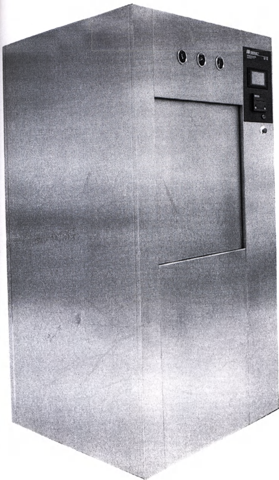
СТЕРИЛИЗАТОР ПАРОВОЙ ГОРИЗОНТАЛЬНЫЙ JSM 70L 1PD. НЕПРОХОДНОЙ (С ОДНОЙ ДВЕРЬЮ) ВИД СПЕРЕДИ (СТОРОНА ЗАГРУЗКИ).
