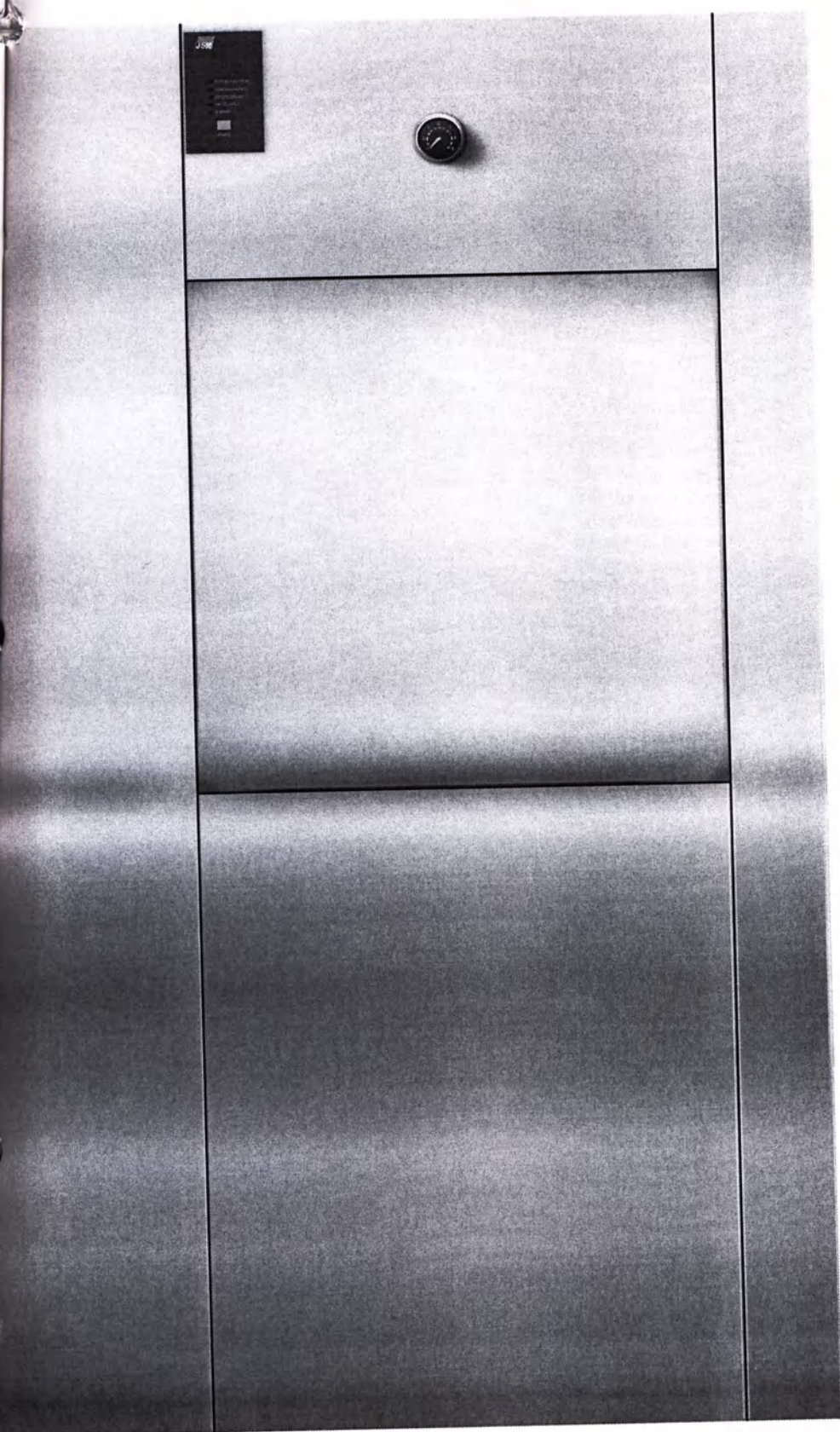
СТЕРИЛИЗАТОР ПАРОВОЙ ГОРИЗОНТАЛЬНЫЙ JSM 70L 2PD ПРОХОДНОЙ (С ДВУМЯ ДВЕРЬМИ). ВИД СЗАДИ (СТОРОНА ВЫГРУЗКИ).
