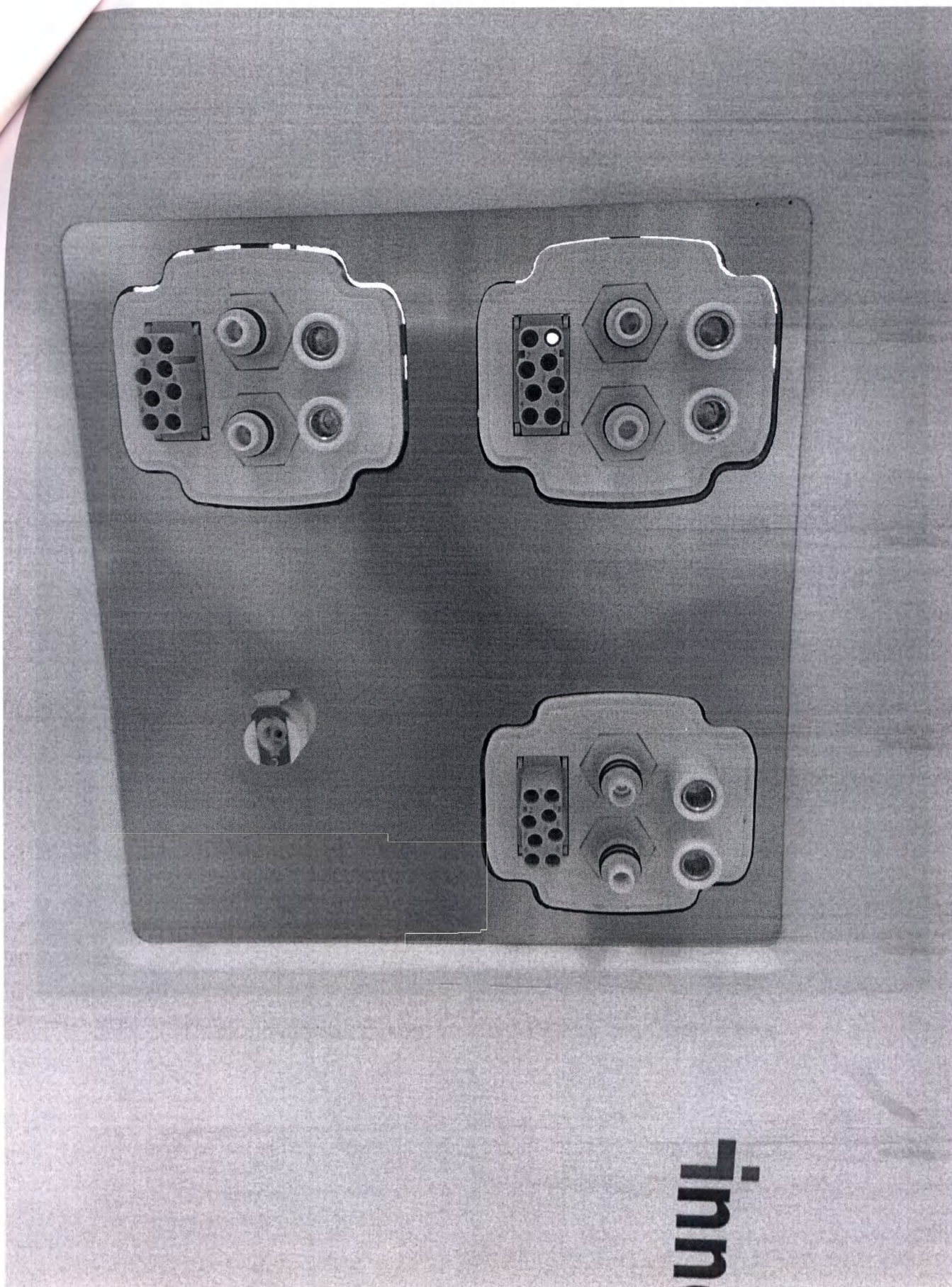
Основной блок. Вид спереди. Панель подключения рукоятей.
