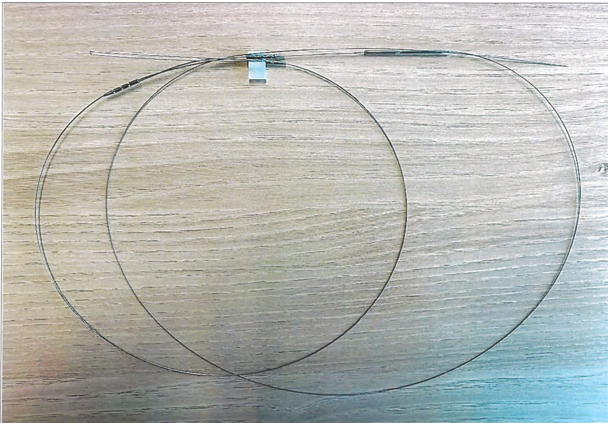
3.1. Устройство для экстракции эндокардиальных электродов LLD EZ, внутренний диаметр электрода 0,015 - 0,023 дюймов.
