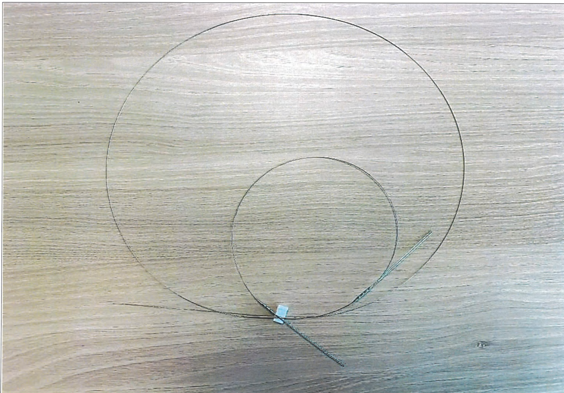
2.1. Устройство для экстракции эндокардиальных электродов LLD E, внутренний диаметр электрода 0,38 - 0,58 дюймов.
