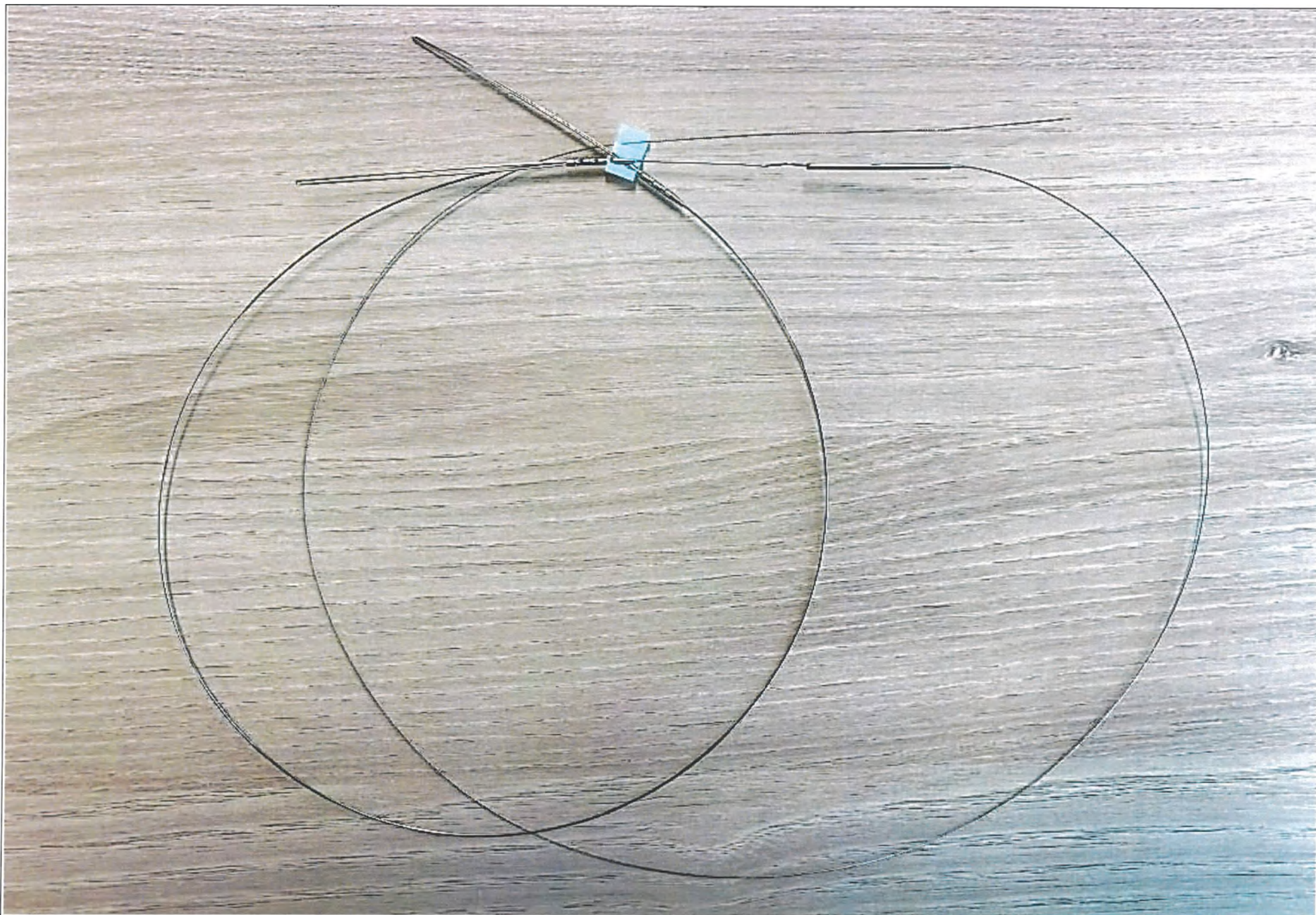
1.1. Устройство для экстракции эндокардиальных электродов LLD № 1, внутренний диаметр электрода 0,013 - 0,016 дюймов.
