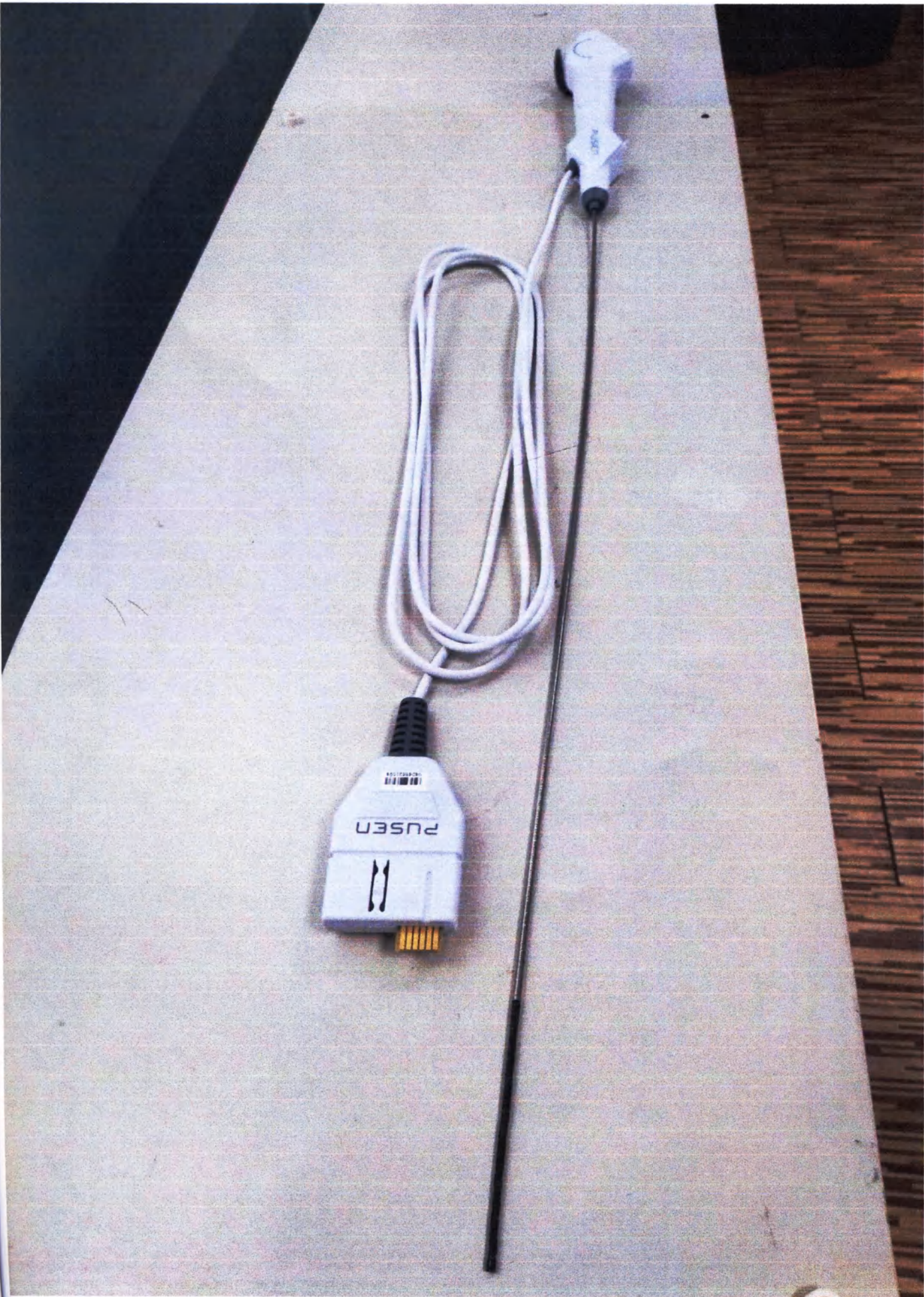
Рисунок 2 - Видеоуретероскоп одноразовый Uscor PU3022
