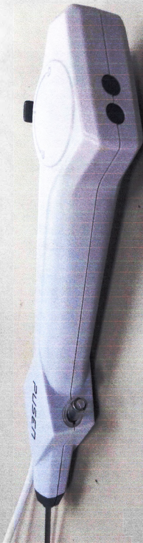
Рисунок 3 – Рукоятка видеoureтероскопа одноразового Uscore PU3022 (без кнопок управления эндоскопом)
