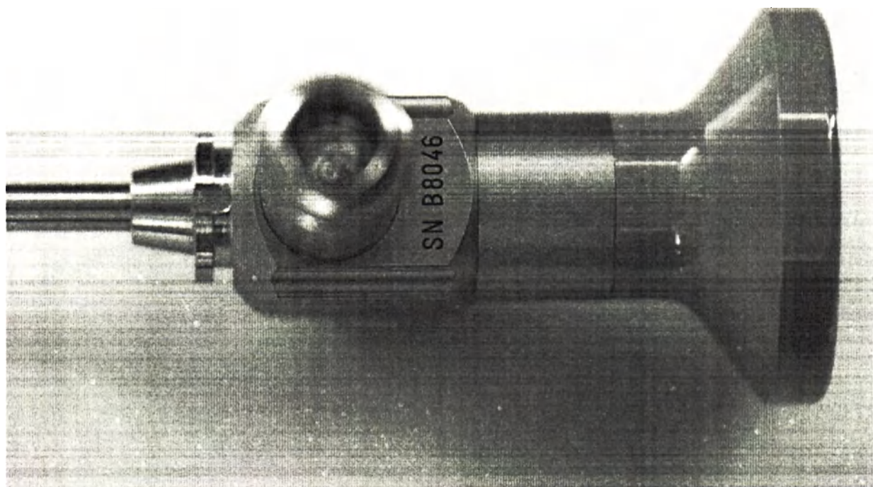
«Эндоскоп Rudolf жесткий», Артроскоп, диаметр 4 мм, длина 175 мм, угол 70°
