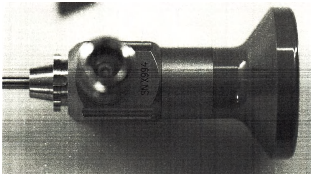
«Эндоскоп Rudolf жесткий», Гистероскоп, диаметр 2,9 мм, длина 302 мм, угол 70°
