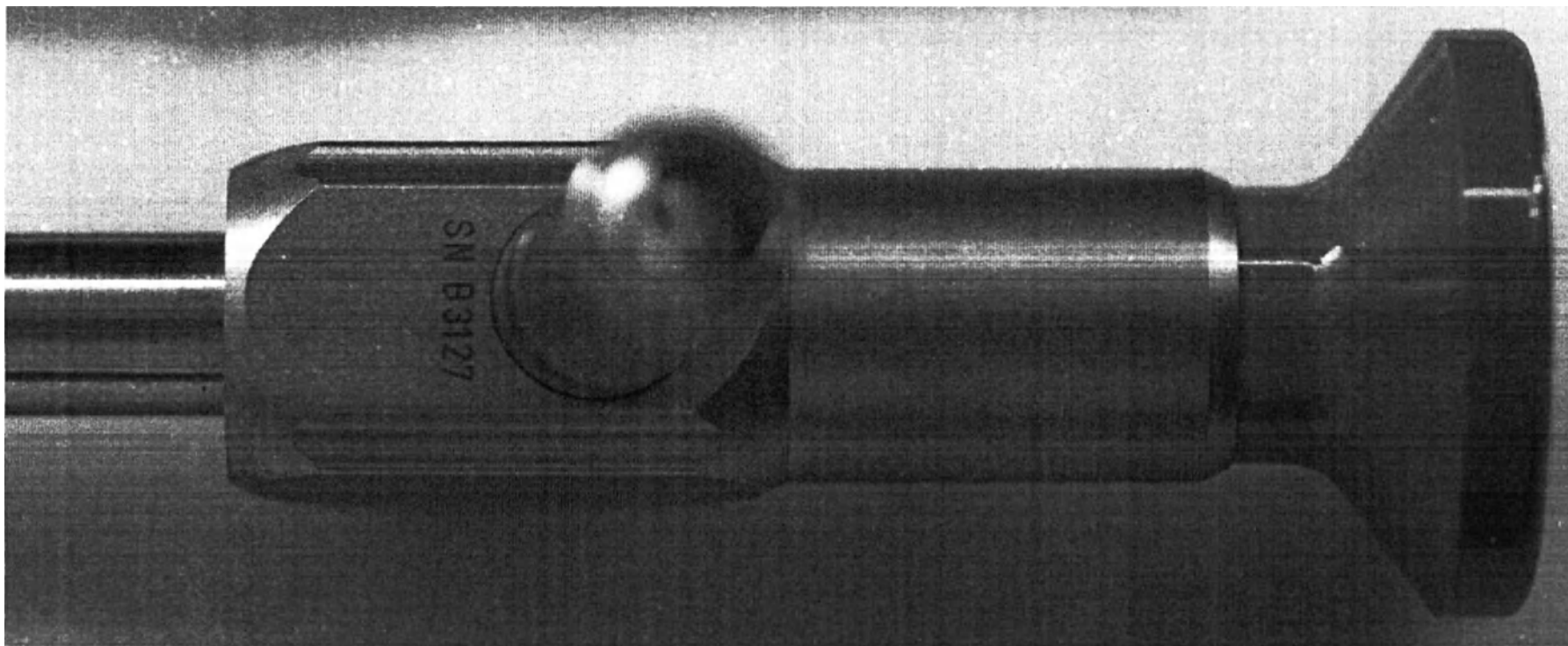
«Эндоскоп Rudolf жесткий», Торакоскоп, диаметр 10,0 мм, длина 170 мм, угол 45°
