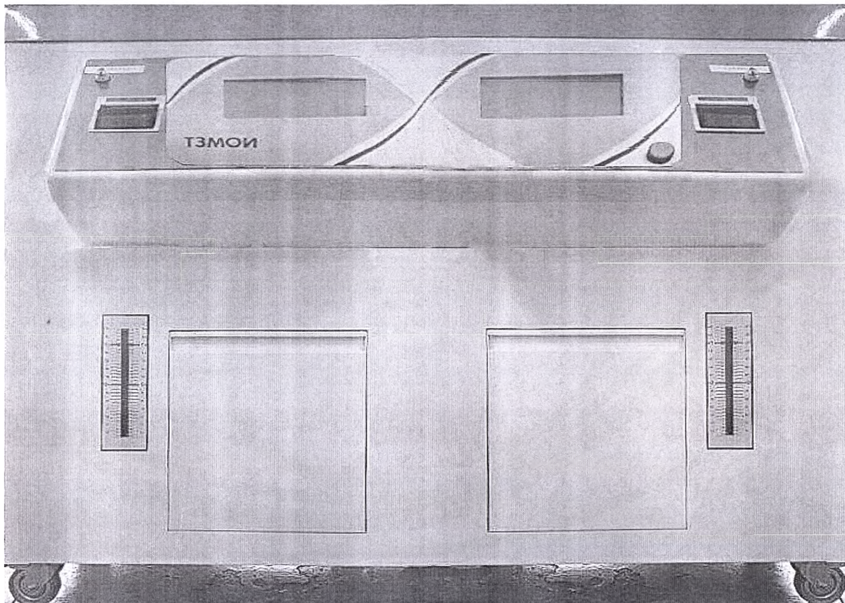
Машина моюще-дезинфицирующая для обработки гибких эндоскопов Флэкс Эндо -2. Внешний вид.
