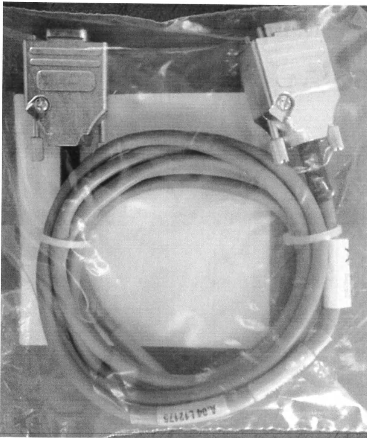
Принадлежности: Кабель последовательного интерфейса RS232, 2м. Общий вид изделия.
