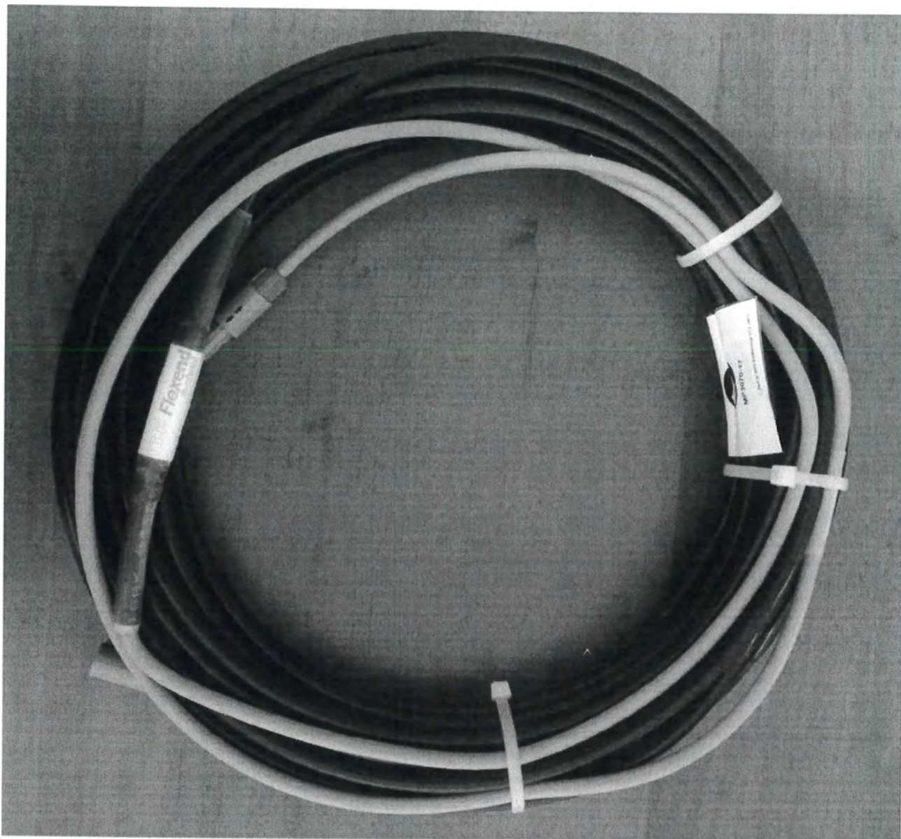
Принадлежности: Удлинительный кабель для стимулирующих импульсов для соединительного модуля, длиной 17 м. Общий вид изделия.
