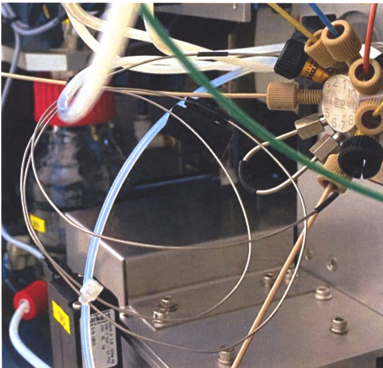
Фотографическое изображение 18 – Петля на 20 мкл (установленная)
