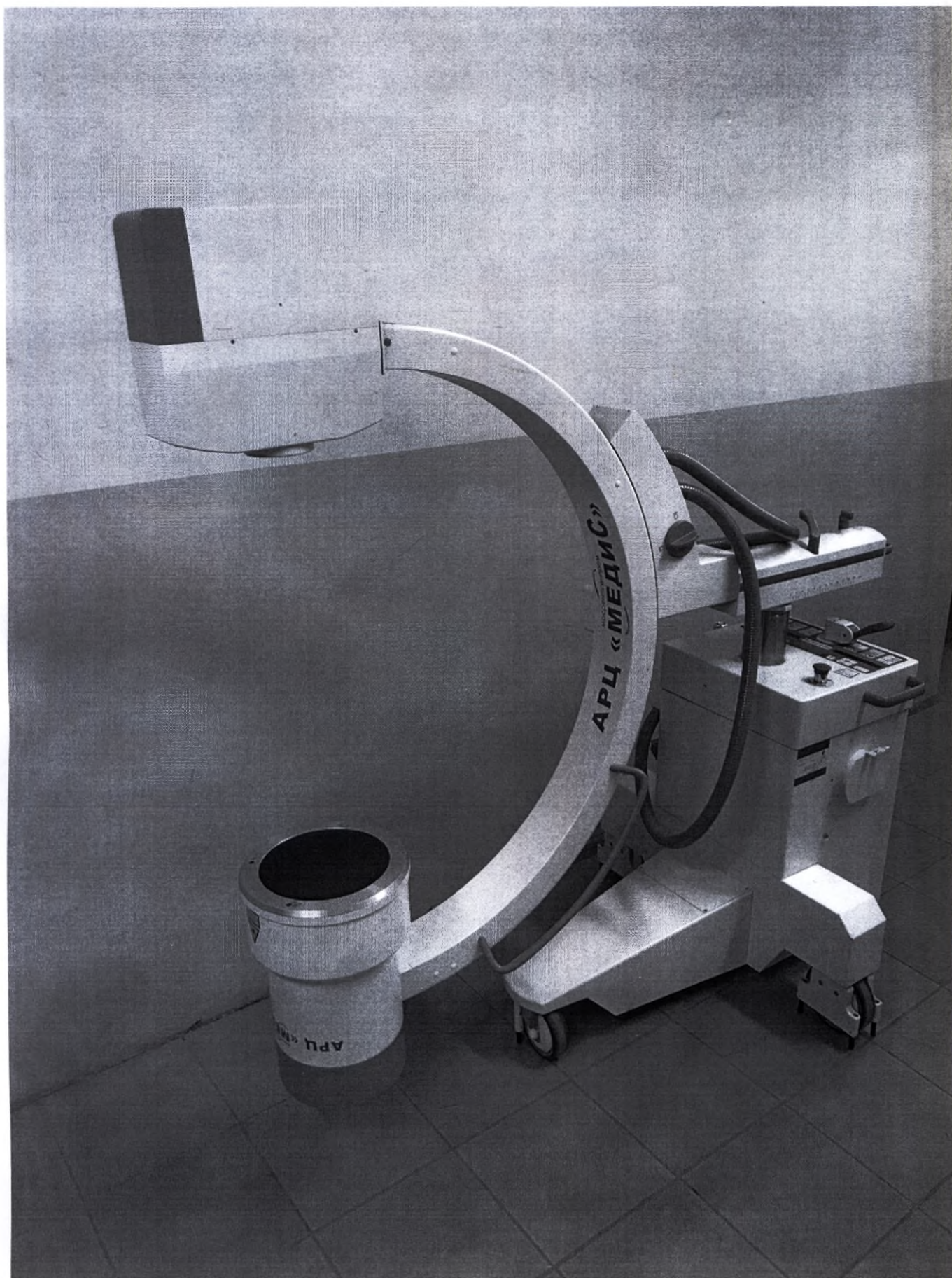
Общий вид медицинского изделия: «Аппарат рентгенодиагностический цифровой «МедиС» (АРЦ «МедиС») по ТУ 26.60.11.113-005-71327975-2018
