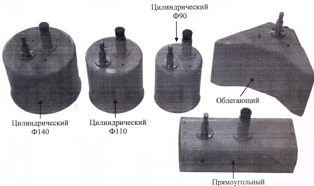
Сменные излучатели
