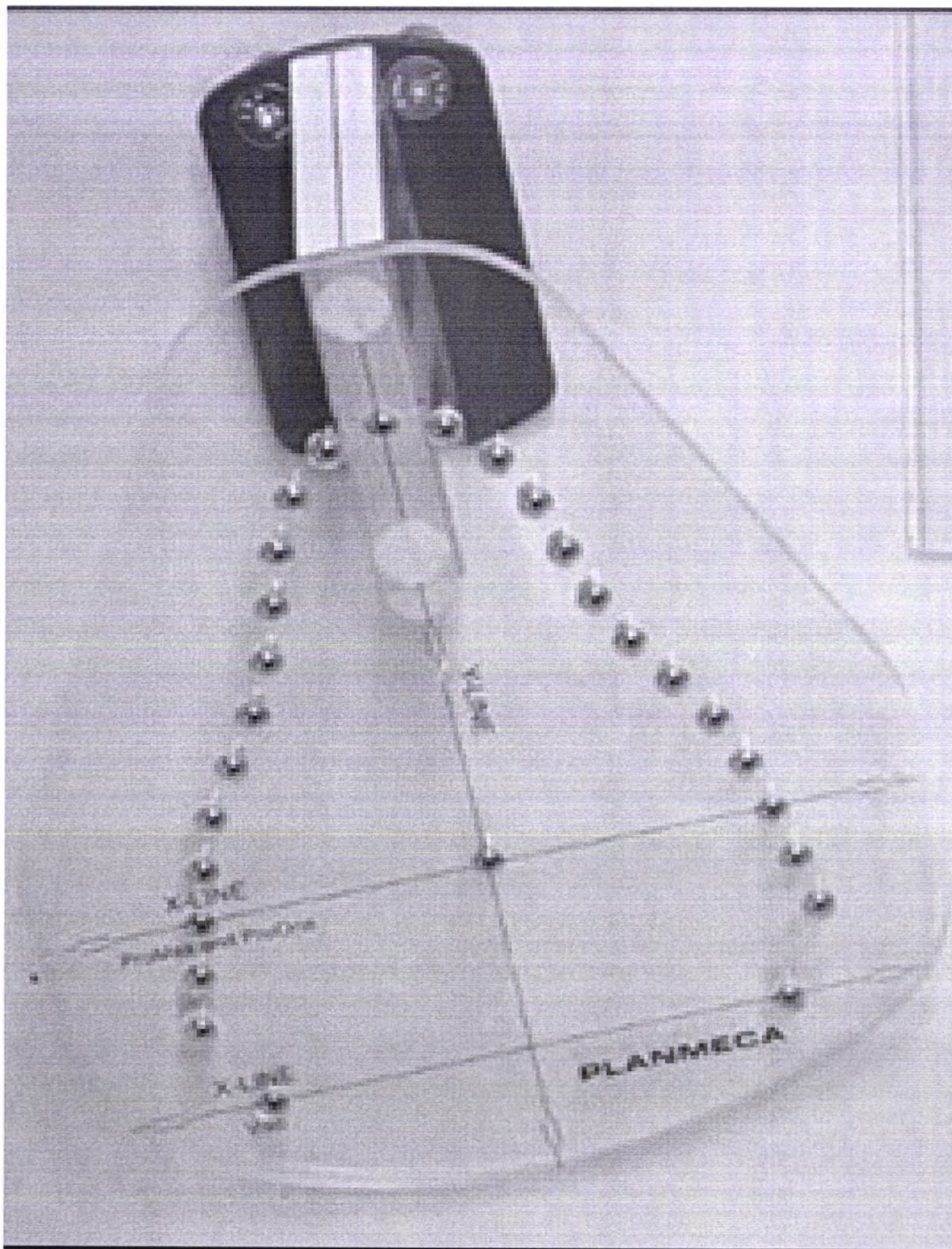
Рис. 37 Фантом шар
