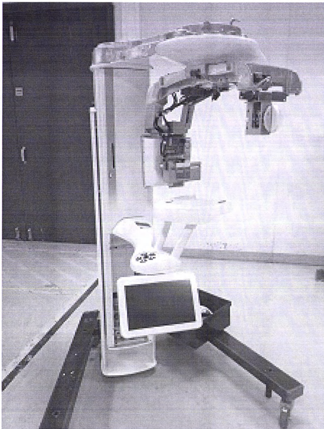
Рис. 1 Установка рентгеновская
