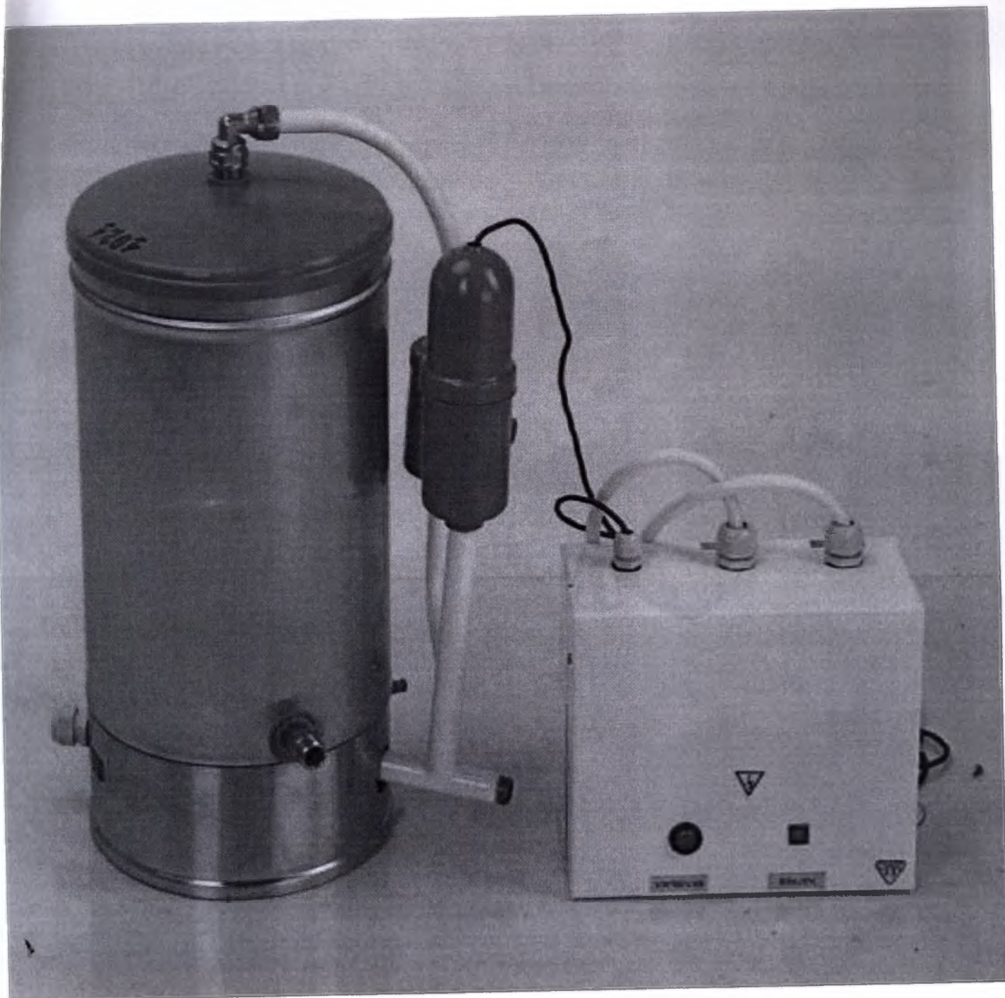
Рисунок 3. Аквадистиллятор электрический ДЭ-4М
