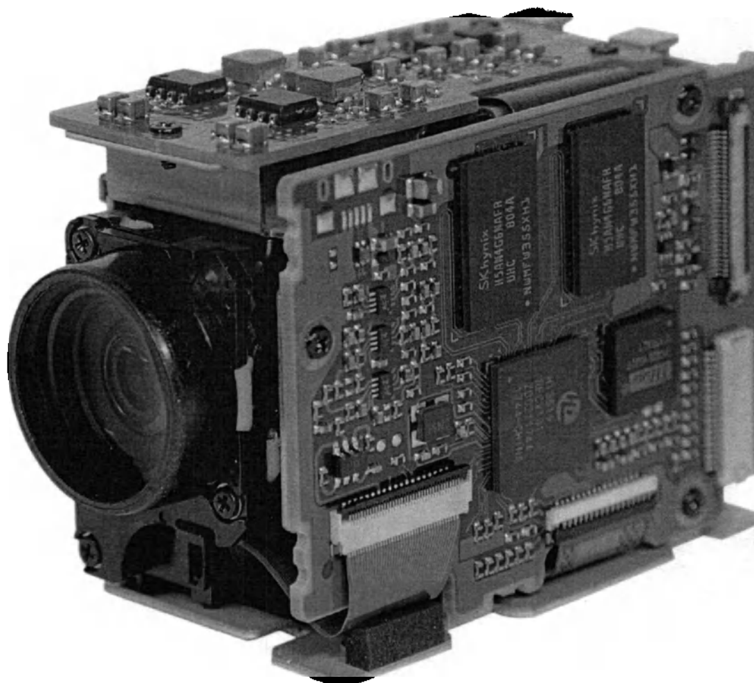
Видеокамера Tamron MP1110M-VC для медицинского изделия Светильники хирургические настенные и потолочные «ЭМАЛЕД» по 9452-013-4665261-2009
