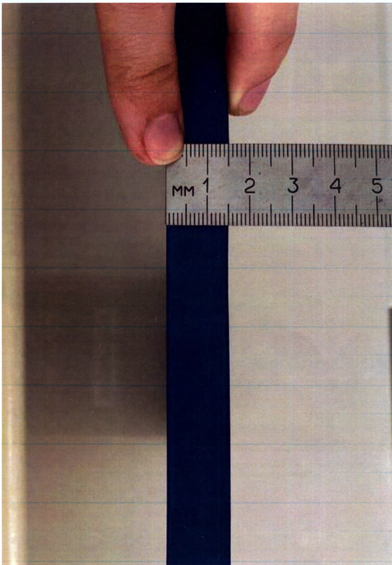
Рисунок 3. Стент коронарный PUT NIY с лекарственным покрытием Сиролимус на системе доставки по ТУ 32.50.22-003-28604018-2019, общий вид с указанием размеров.
