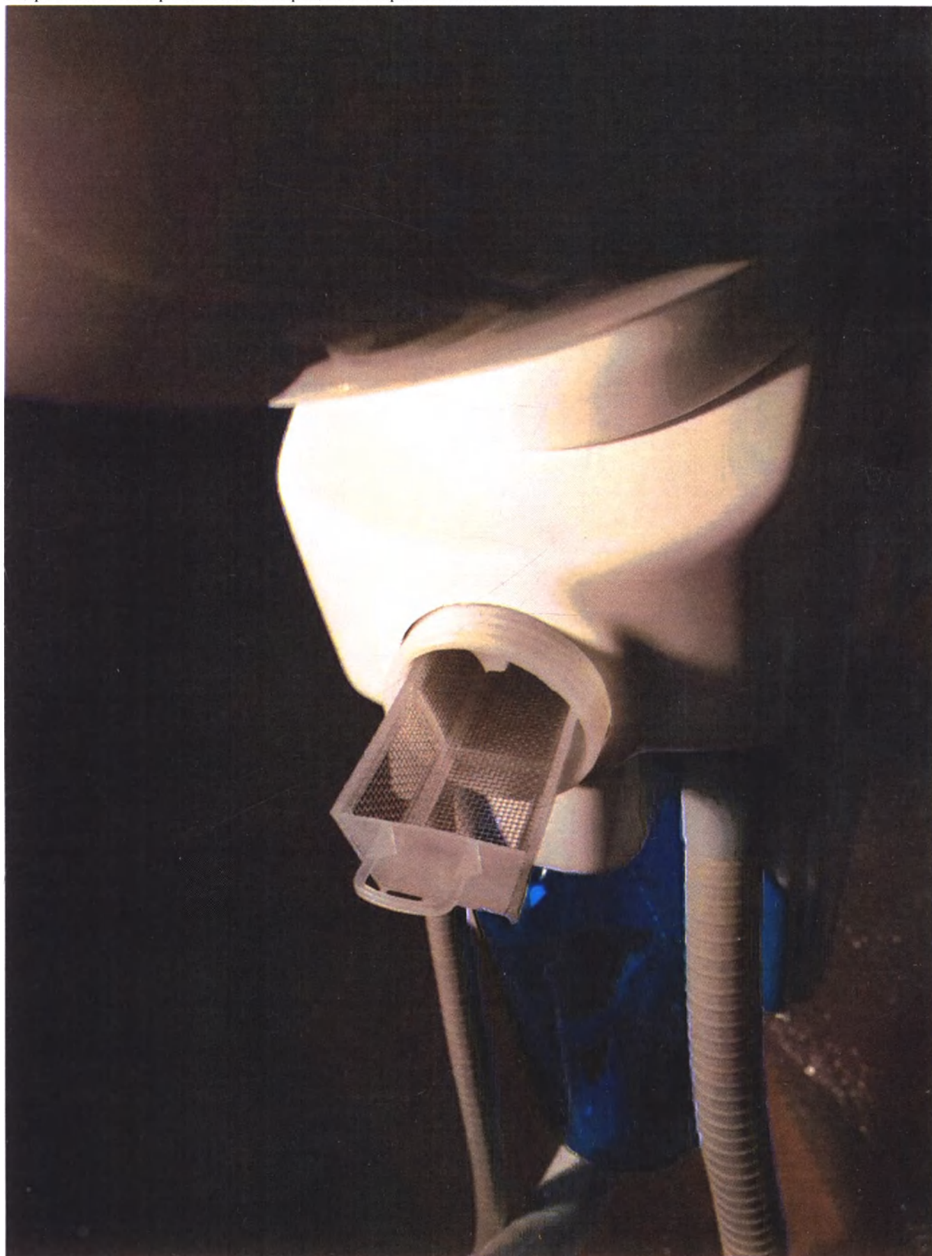
Гидроблок. Фильтр системы аспирации в открытом положении
