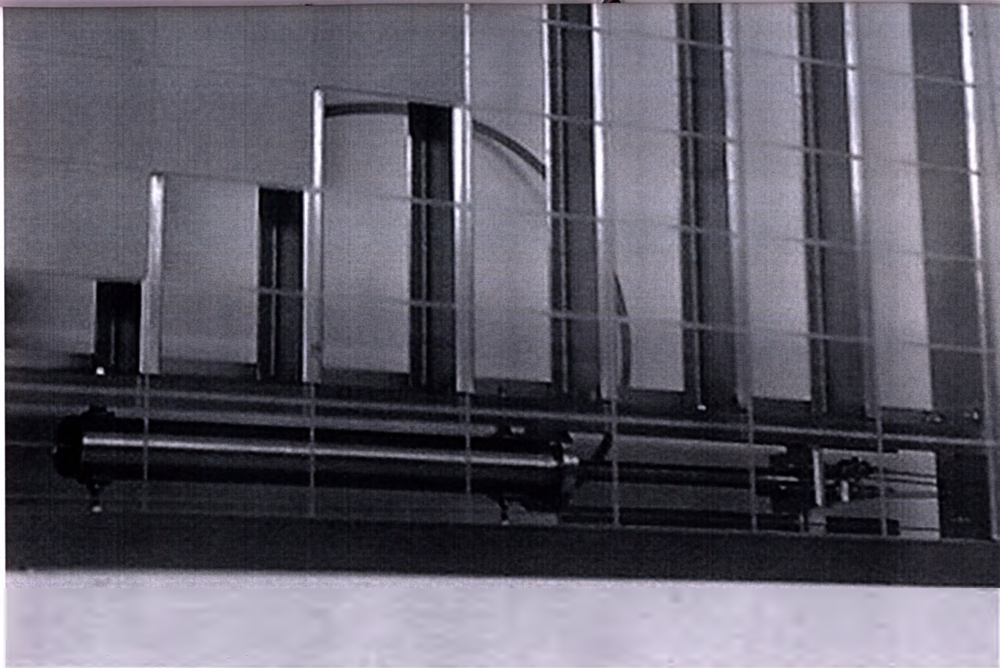
Гидравлическая установка: - поршень, длина 3500мм, диаметр 23 см
