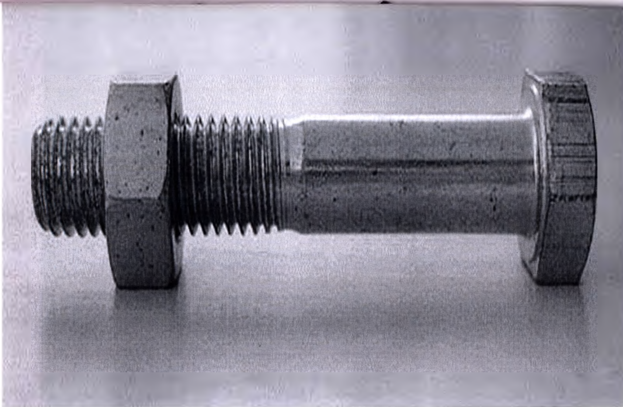
Фальшпол (дно), регулируемый по высоте: - болты M12x60;- гайки M12
