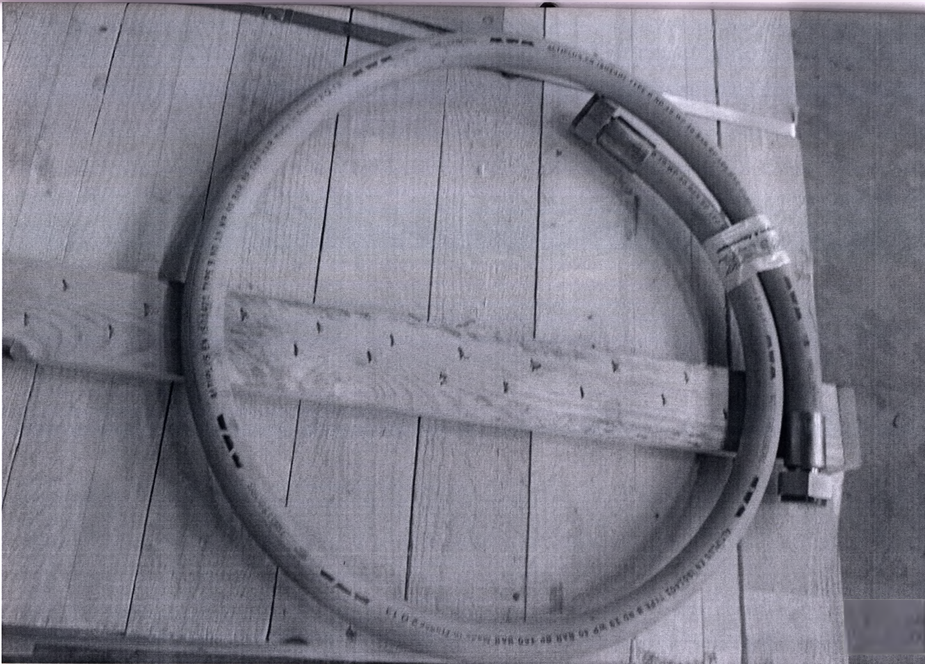
Гидравлическая установка: - шланг высокого давления, длина 10 м
