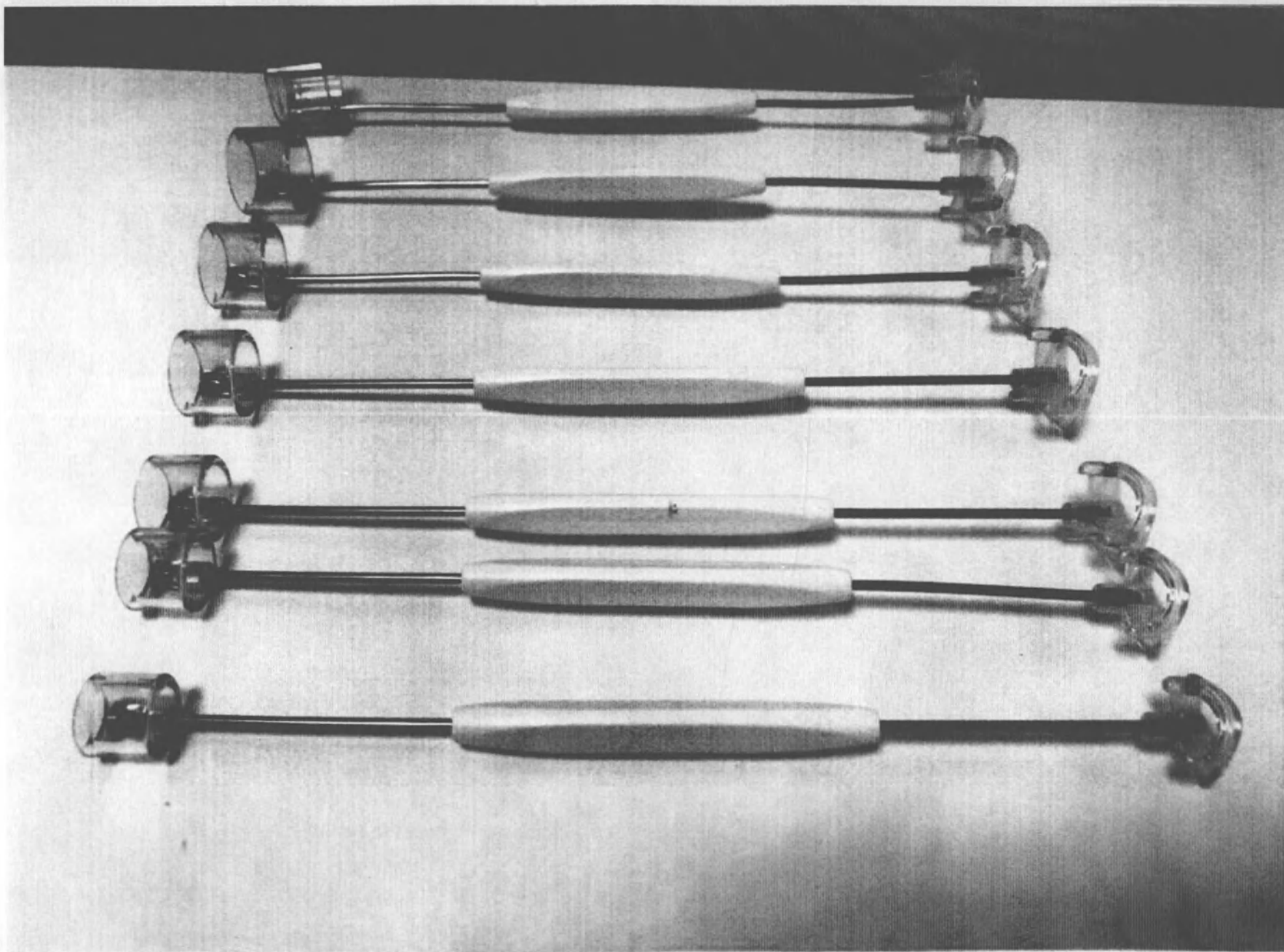
Рисунок 13. Измеритель диаметра клапана Avalus
