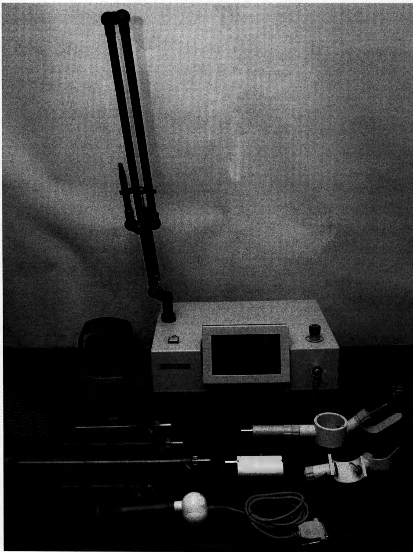
Общий вид аппарата лазерного медицинского АЛМ-30-01 «ЛГ Мед-1» с принадлежностями, необходимыми для применения по назначению
