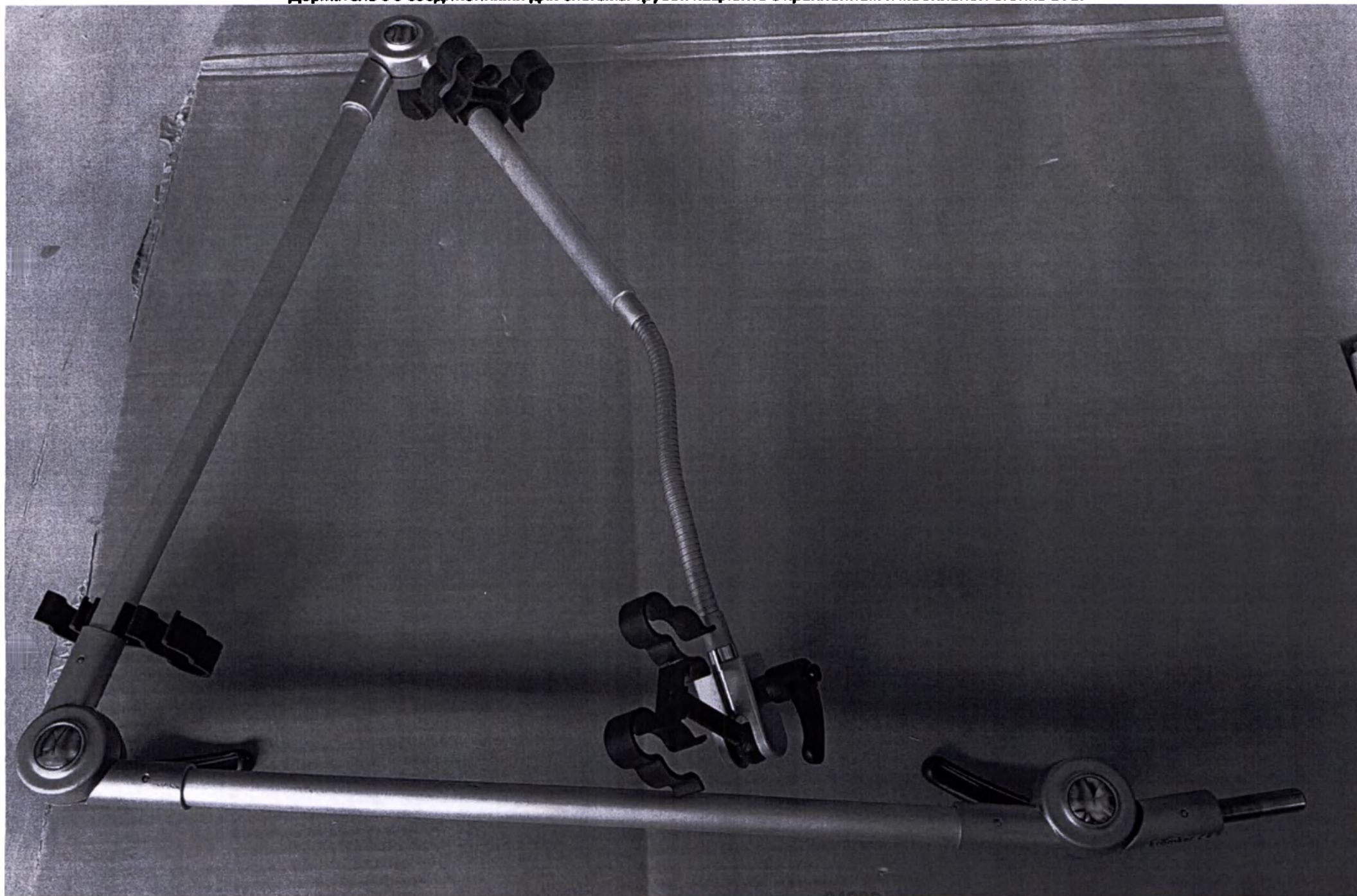
Держатель с 3 соединениями для системы трубок пациента с креплением к мобильной стойке EVE.
