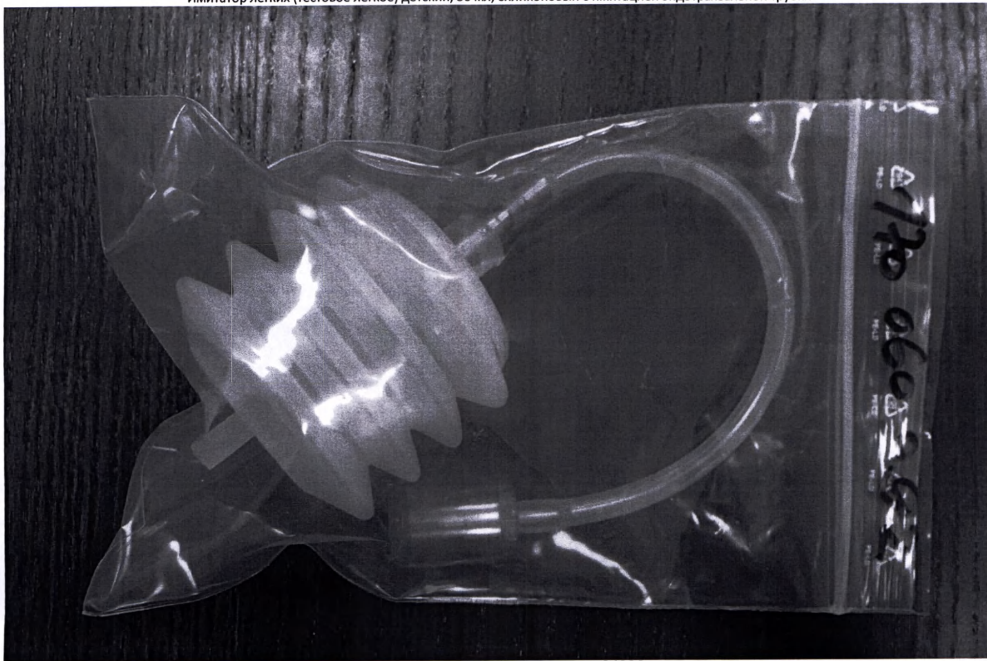
Имитатор легких (тестовое легкое) детский, 30 мл, силиконовый с имитацией эндотрахеальной трубки
