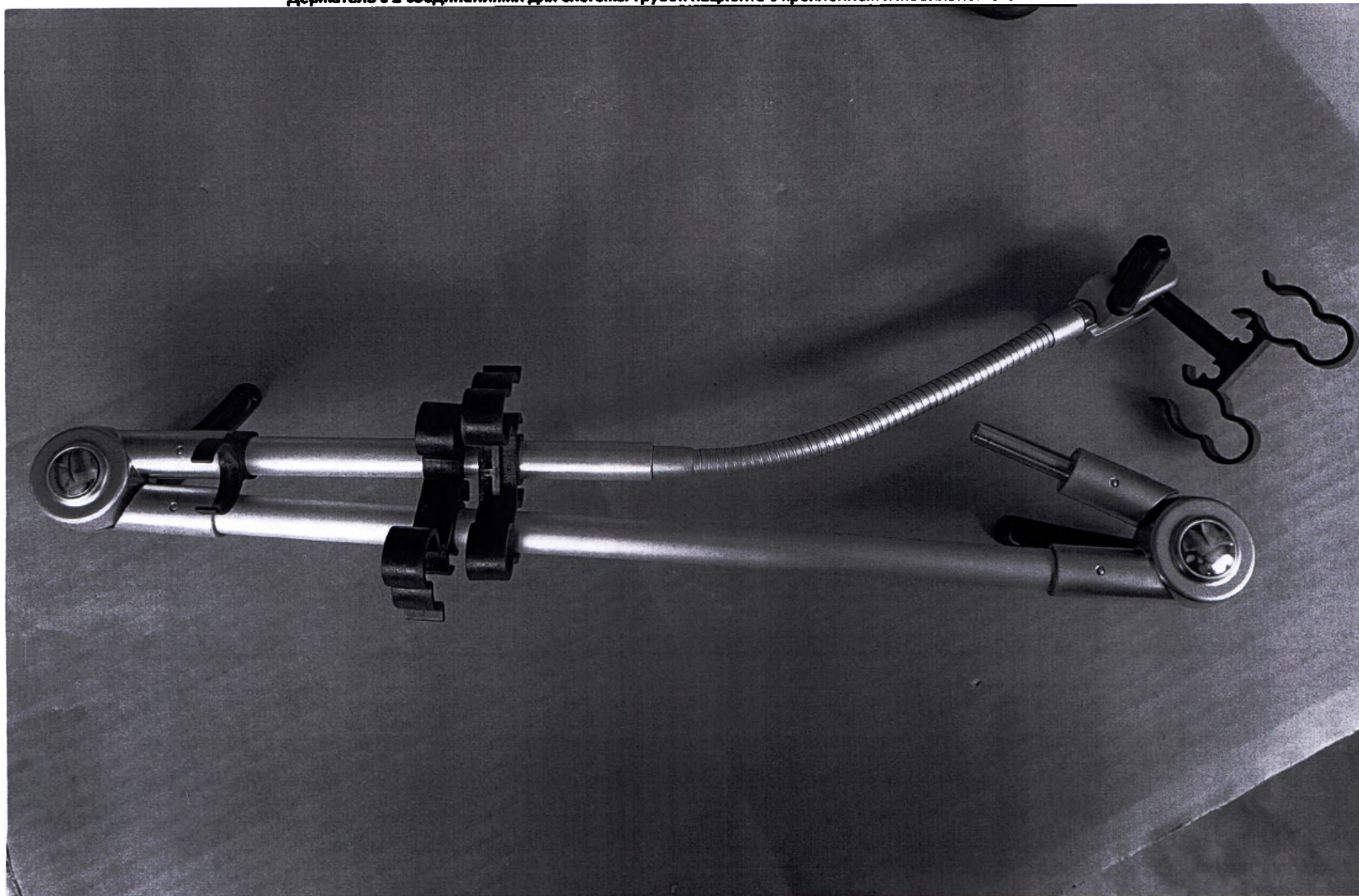
Держатель с 2 соединениями для системы трубок пациента с креплением к мобильной стойке EVE.
