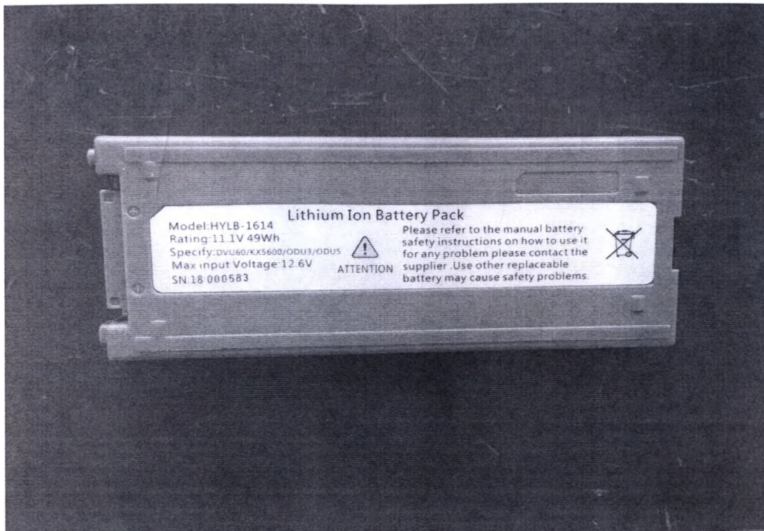
Аккумуляторная батарея
