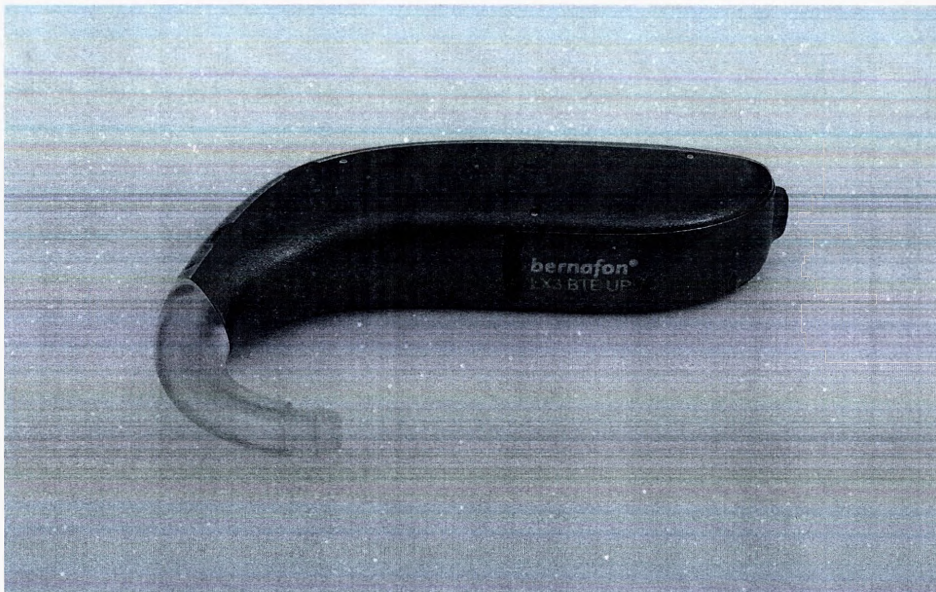
Аппарат слуховой электронный цифровой программируемый воздушного звукопроводения заушного типа LEOX 3 BTE UP (LX3 BTE UP)
