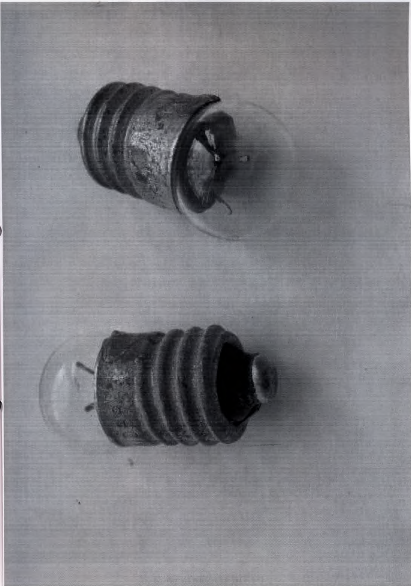
4. Лампа МН 26-0,12-1
